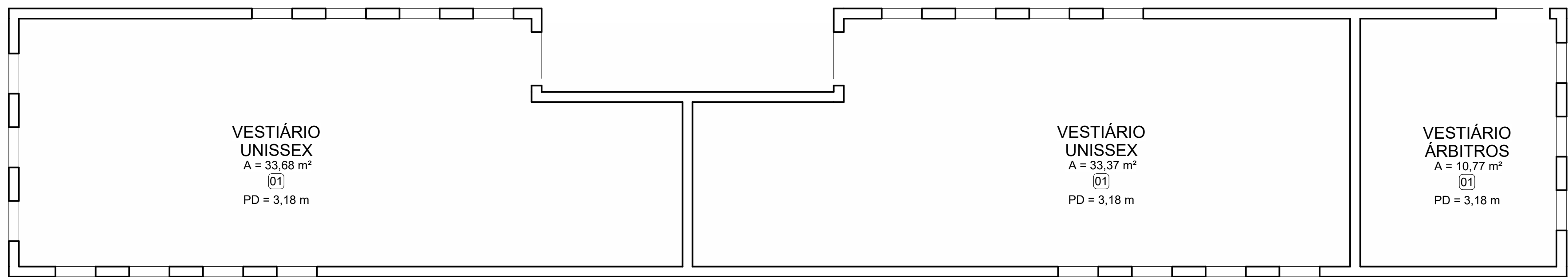
3 PLANTA DE FORRO - VESTIÁRIO ESCALA: 1 : 50
