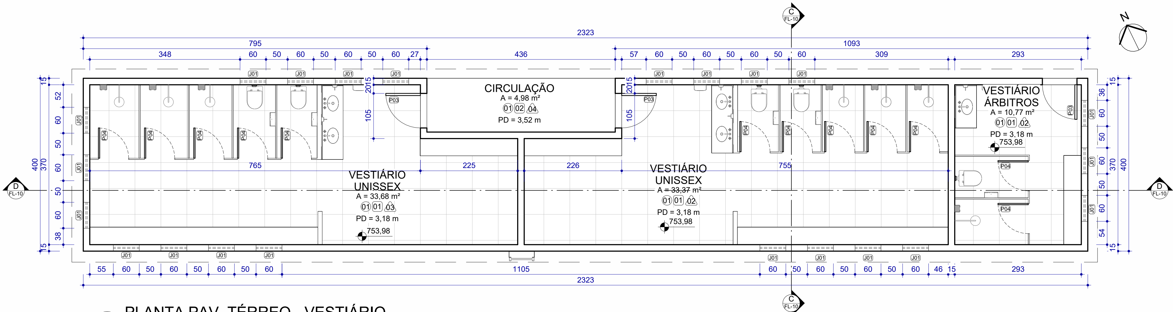
5 PLANTA PAV. TÉRREO - VESTIÁRIO
