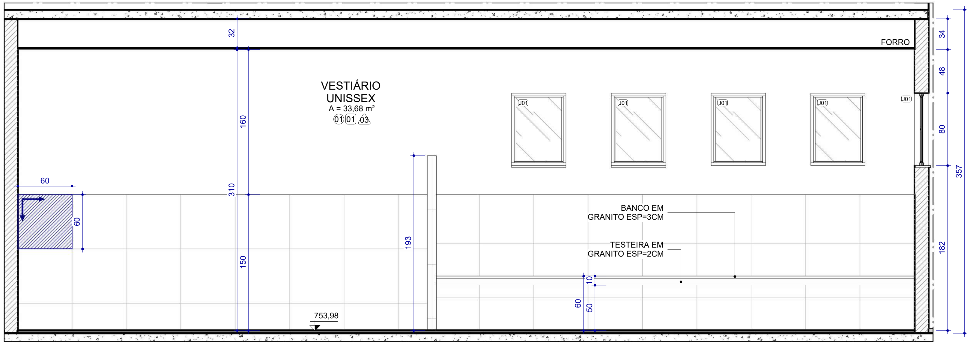
C REFORMA - ELEVAÇÃO C - VESTIÁRIO UNISSEX ESCALA: 1 : 25
