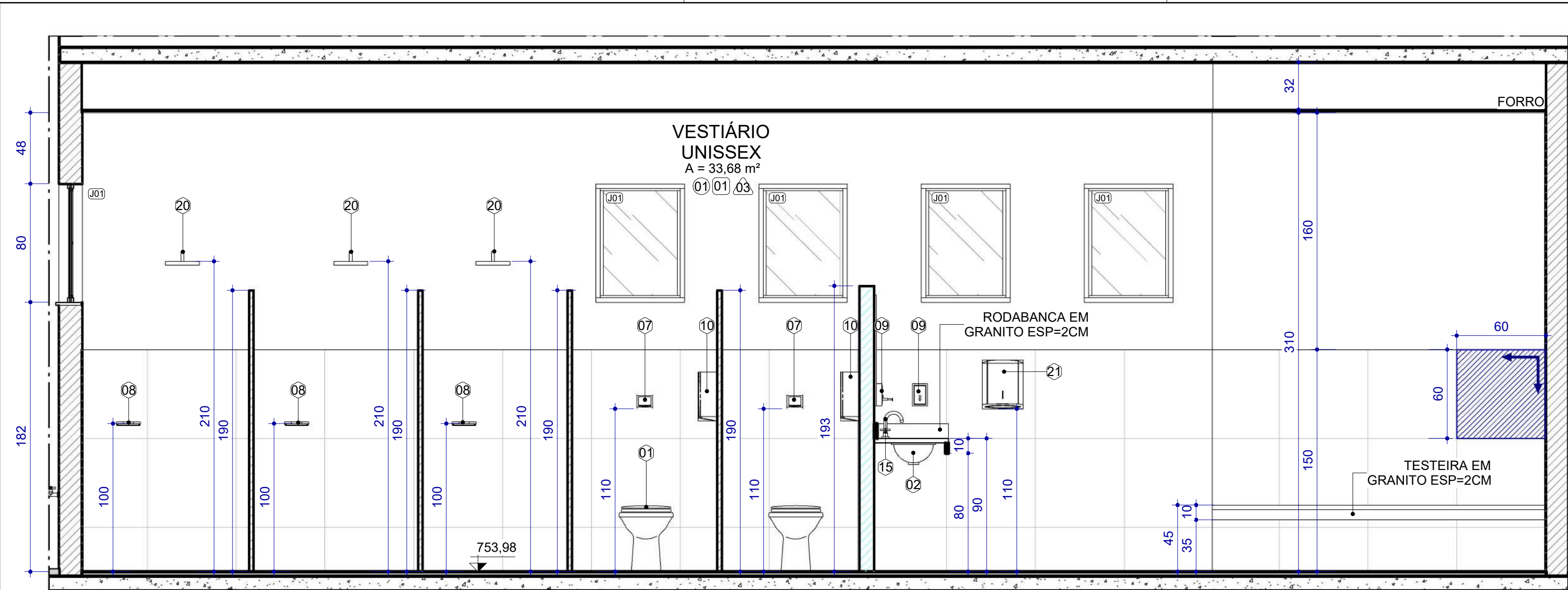
A REFORMA - ELEVAÇÃO A - VESTIÁRIO UNISSEX ESCALA: 1 : 25
