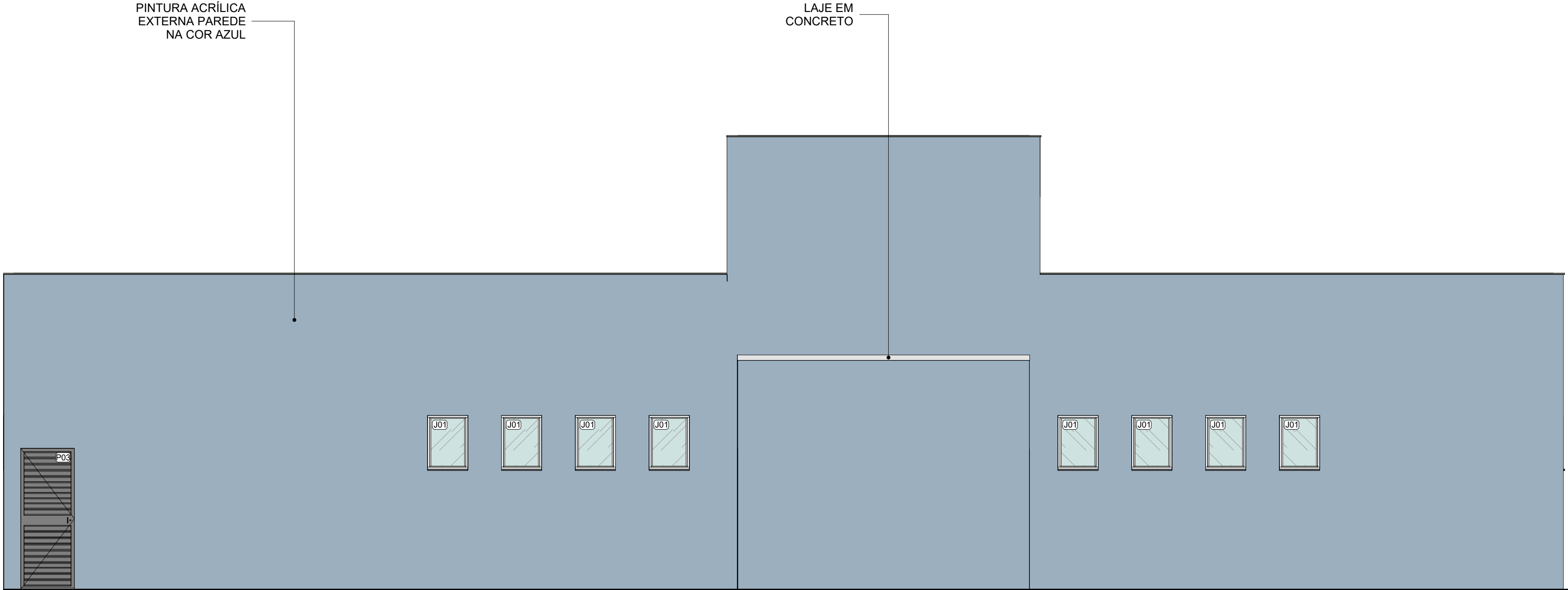
1 FACHADA FRONTAL - VESTIÁRIO ESCALA: 1 : 50
