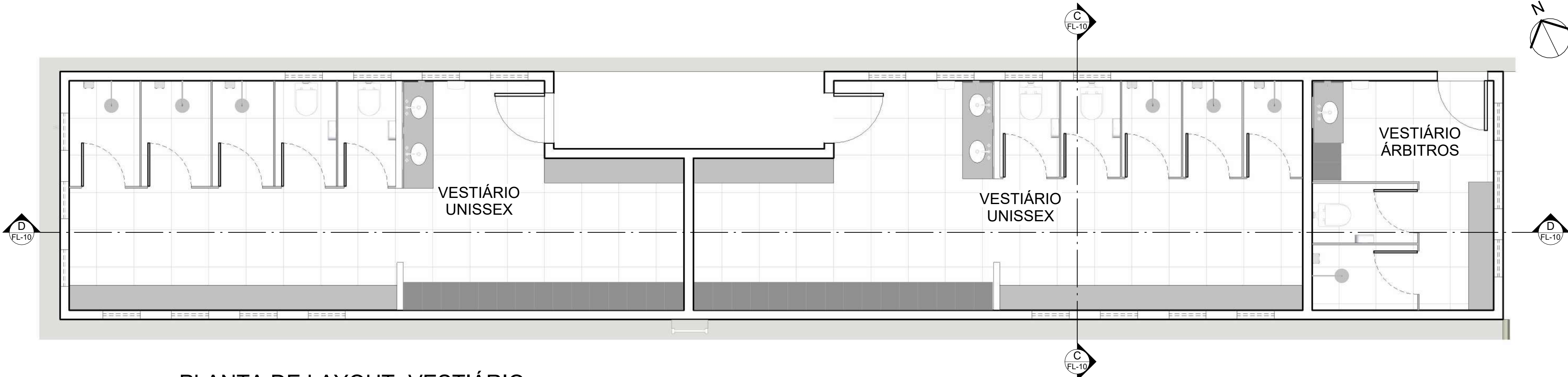
7 PLANTA DE LAYOUT- VESTIÁRIO
