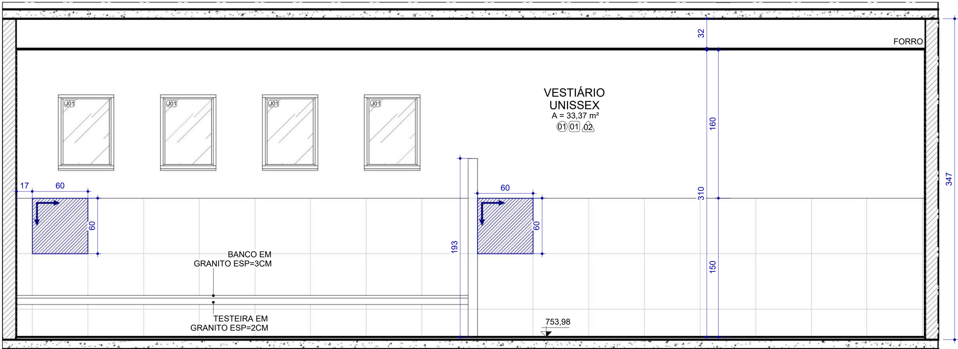
A REFORMA - ELEVAÇÃO C - VESTIÁRIO
