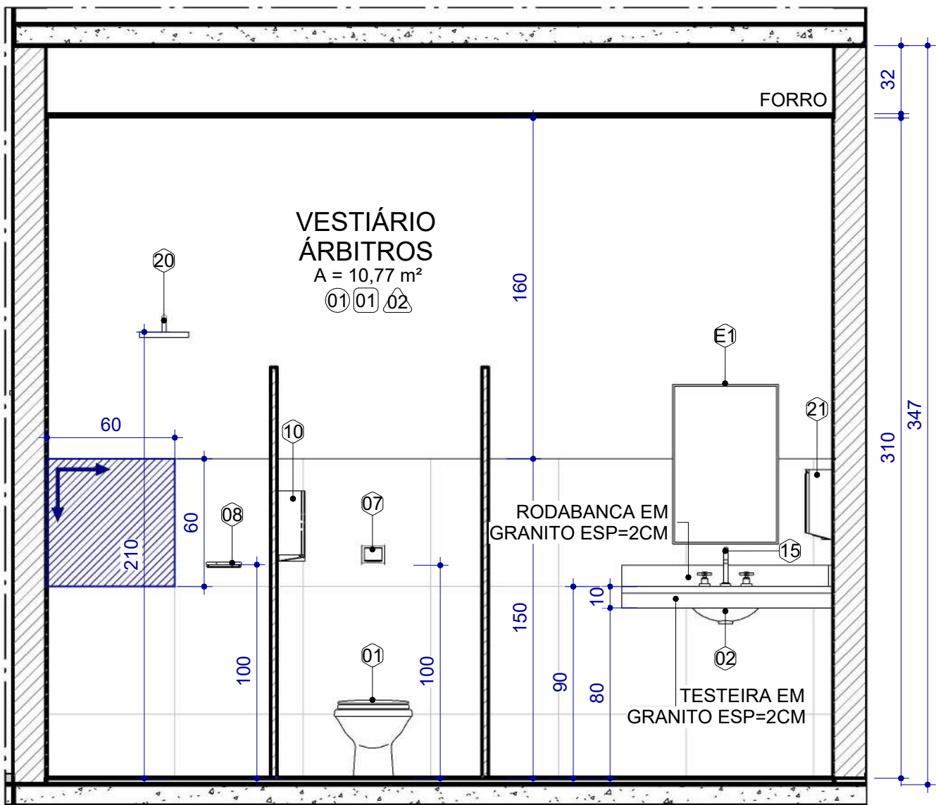
E REFORMA - ELEVAÇÃO D - VESTIÁRIO ÁRBITROS
