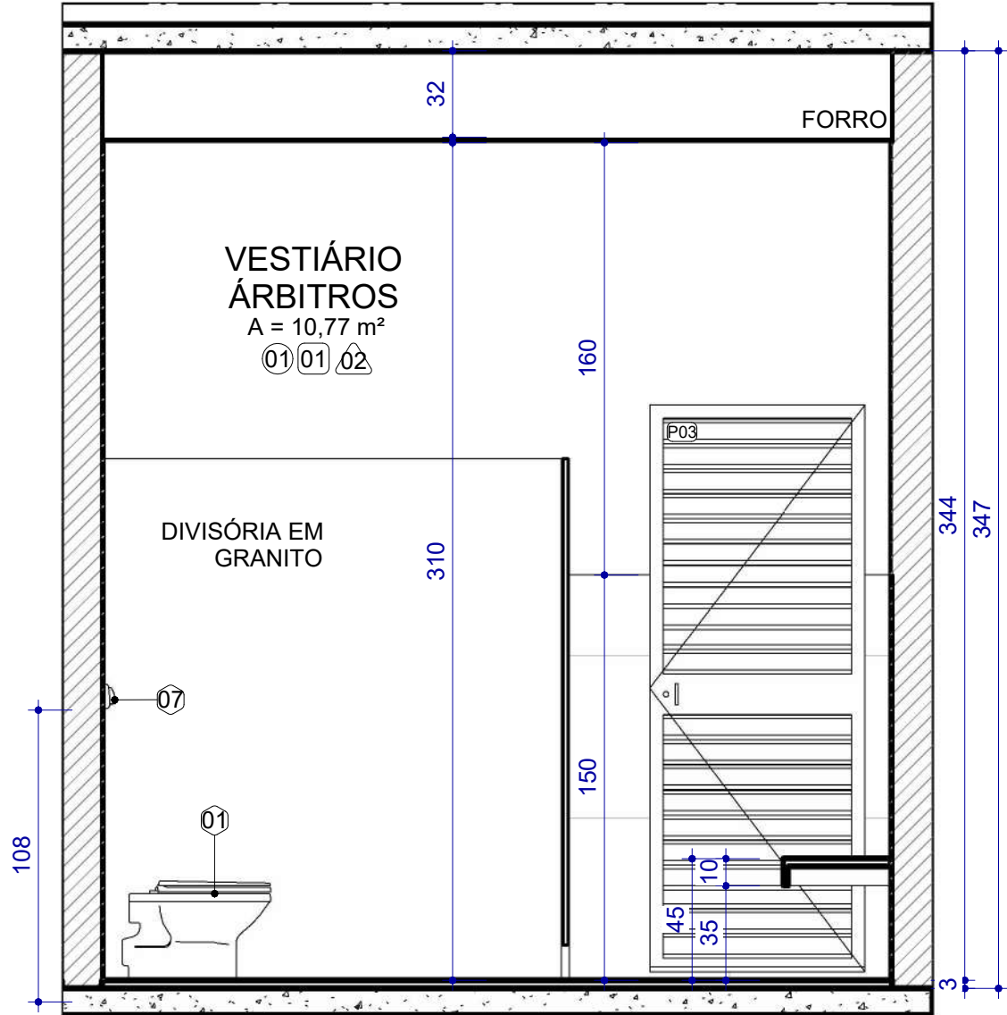
B REFORMA - ELEVAÇÃO A - VESTIÁRIO ÁRBITROS
