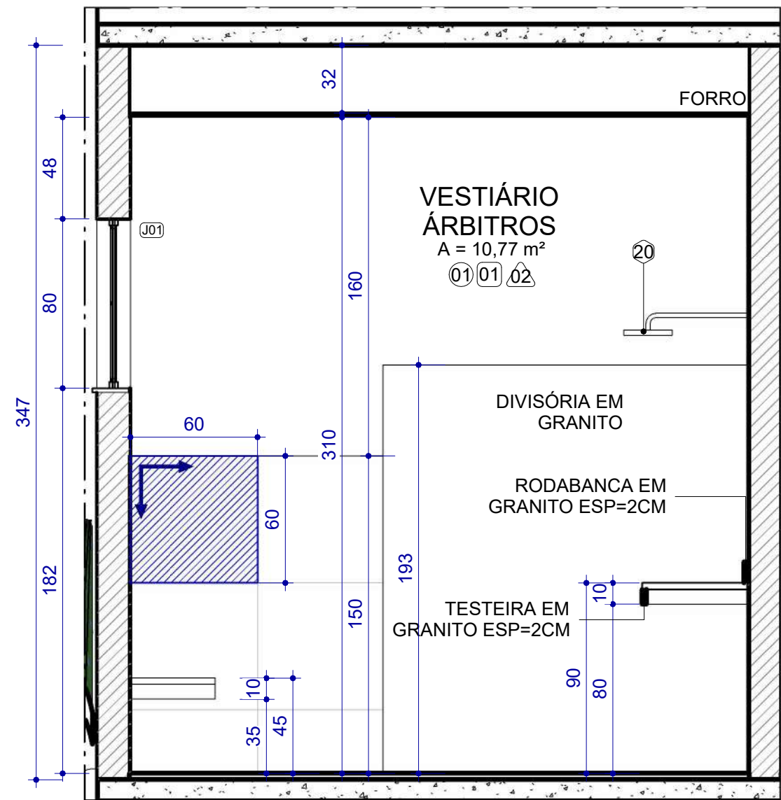
D REFORMA - ELEVAÇÃO C - VESTIÁRIO ÁRBITROS
