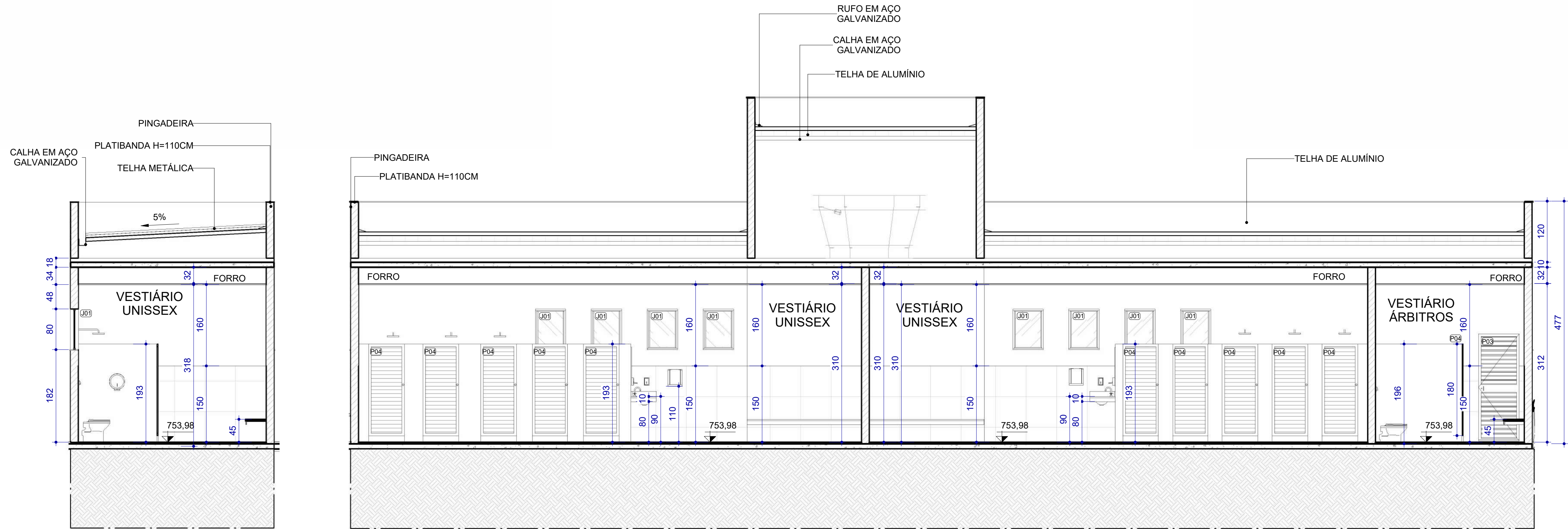
C NOVA CONSTRUÇÃO VESTIÁRIO - CORTE CC ESCALA: 1 : 50
