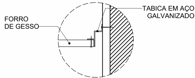
5 DET. TABICA FORRO DE GESSO ESCALA: 1 : 5
