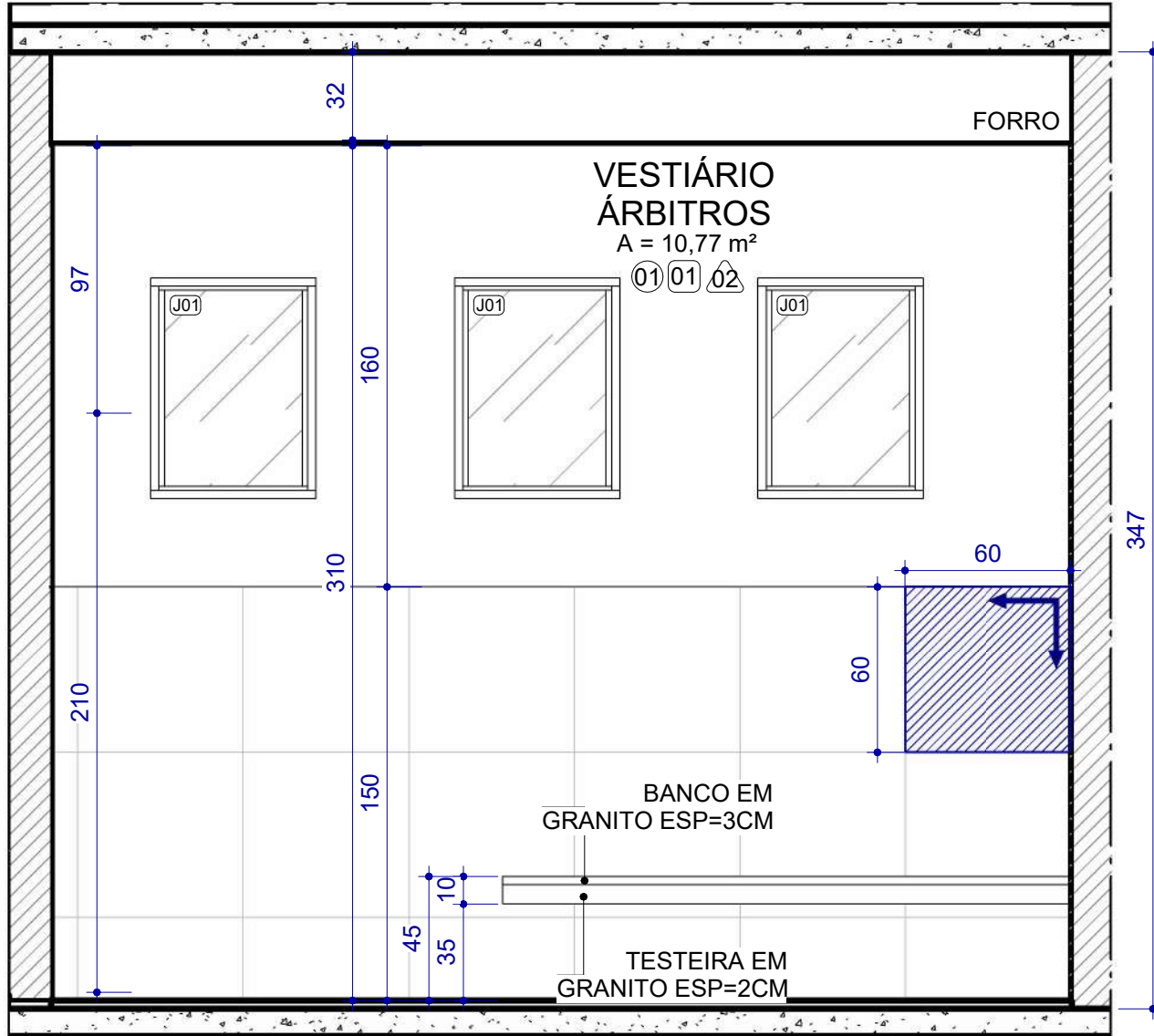
C REFORMA - ELEVAÇÃO B - VESTIÁRIO ÁRBITROS
