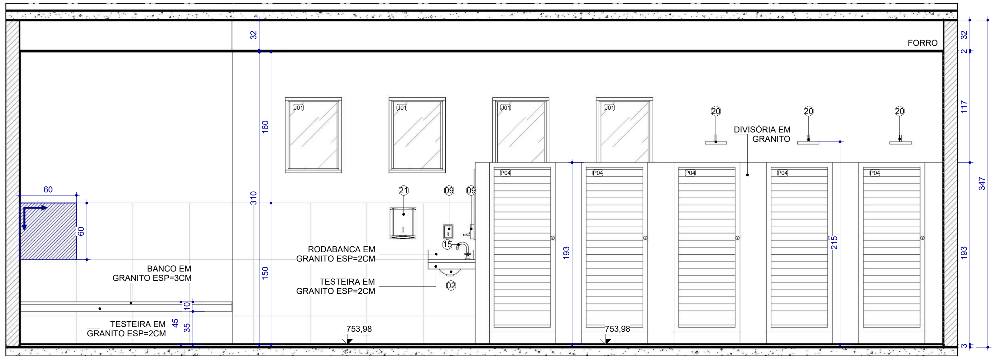
E REFORMA - ELEVAÇÃO A - VESTIÁRIO ESCALA: 1 : 25
