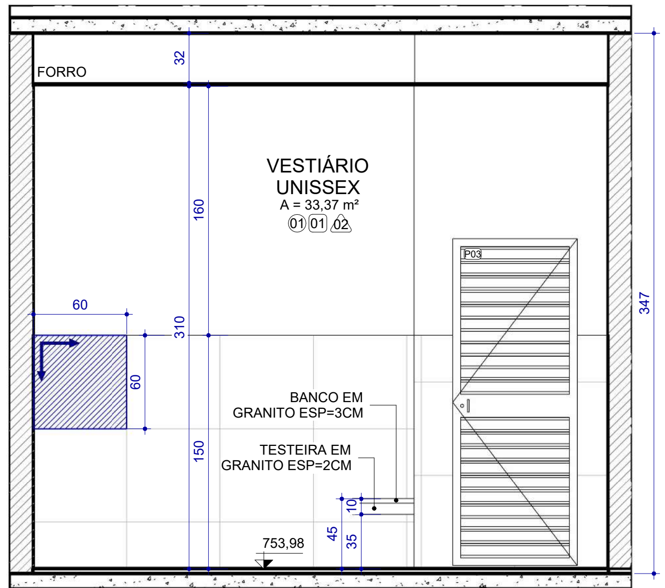
F REFORMA - ELEVAÇÃO D - VESTIÁRIO ESCALA: 1 : 25
