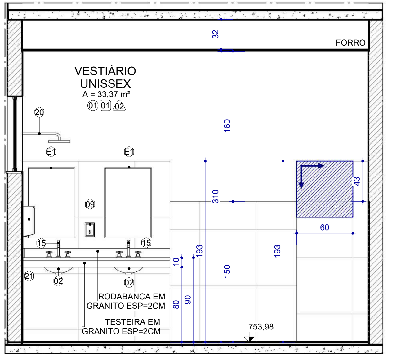
D REFORMA - ELEVAÇÃO B - VESTIÁRIO ESCALA: 1 : 25
