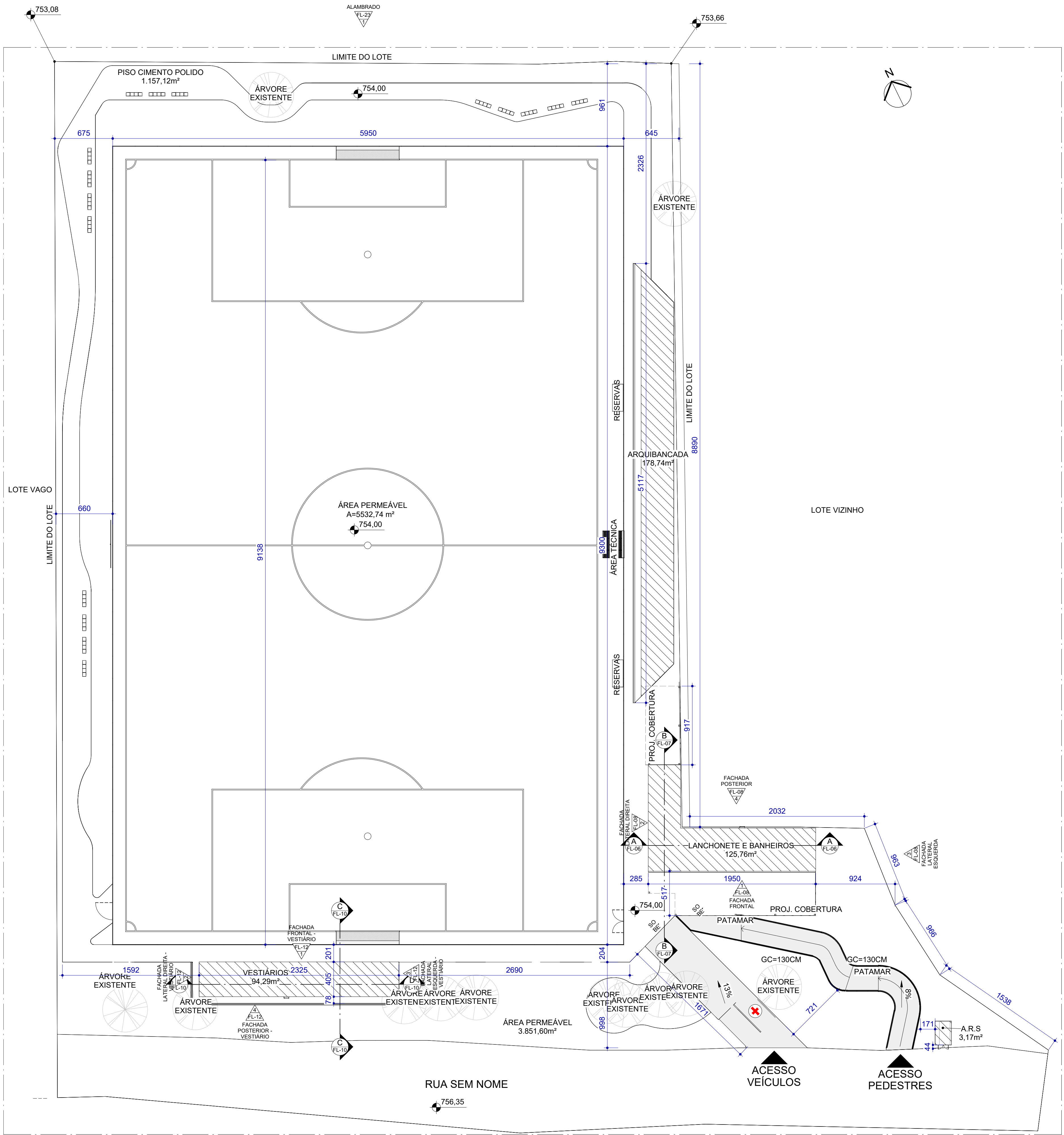
1 PLANTA DE IMPLANTAÇÃO ESCALA: 1 : 250
