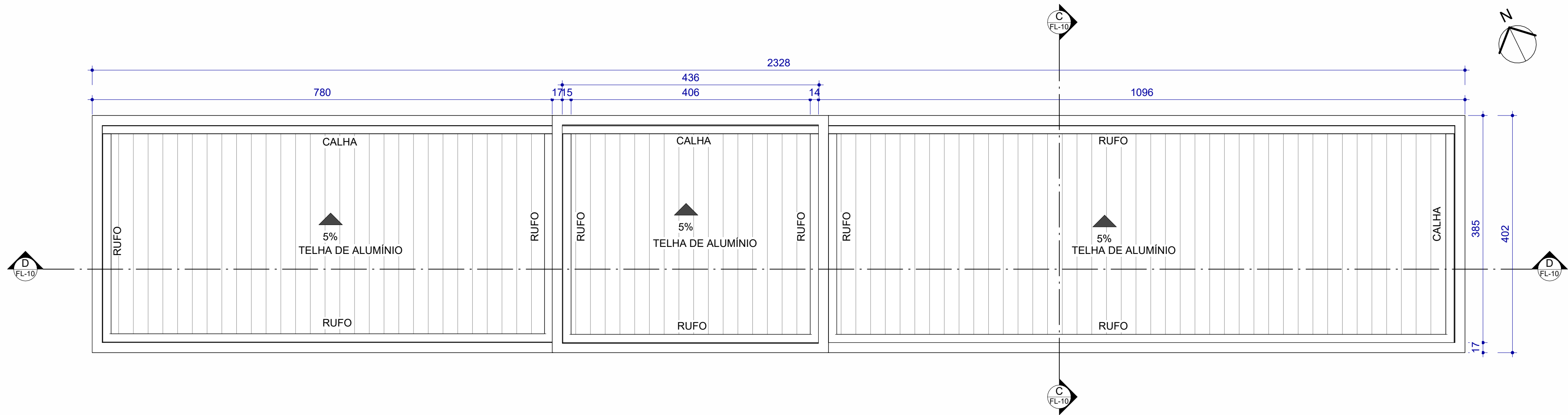
4 PLANTA DE COBERTURA - VESTIÁRIO ESCALA: 1 : 50
