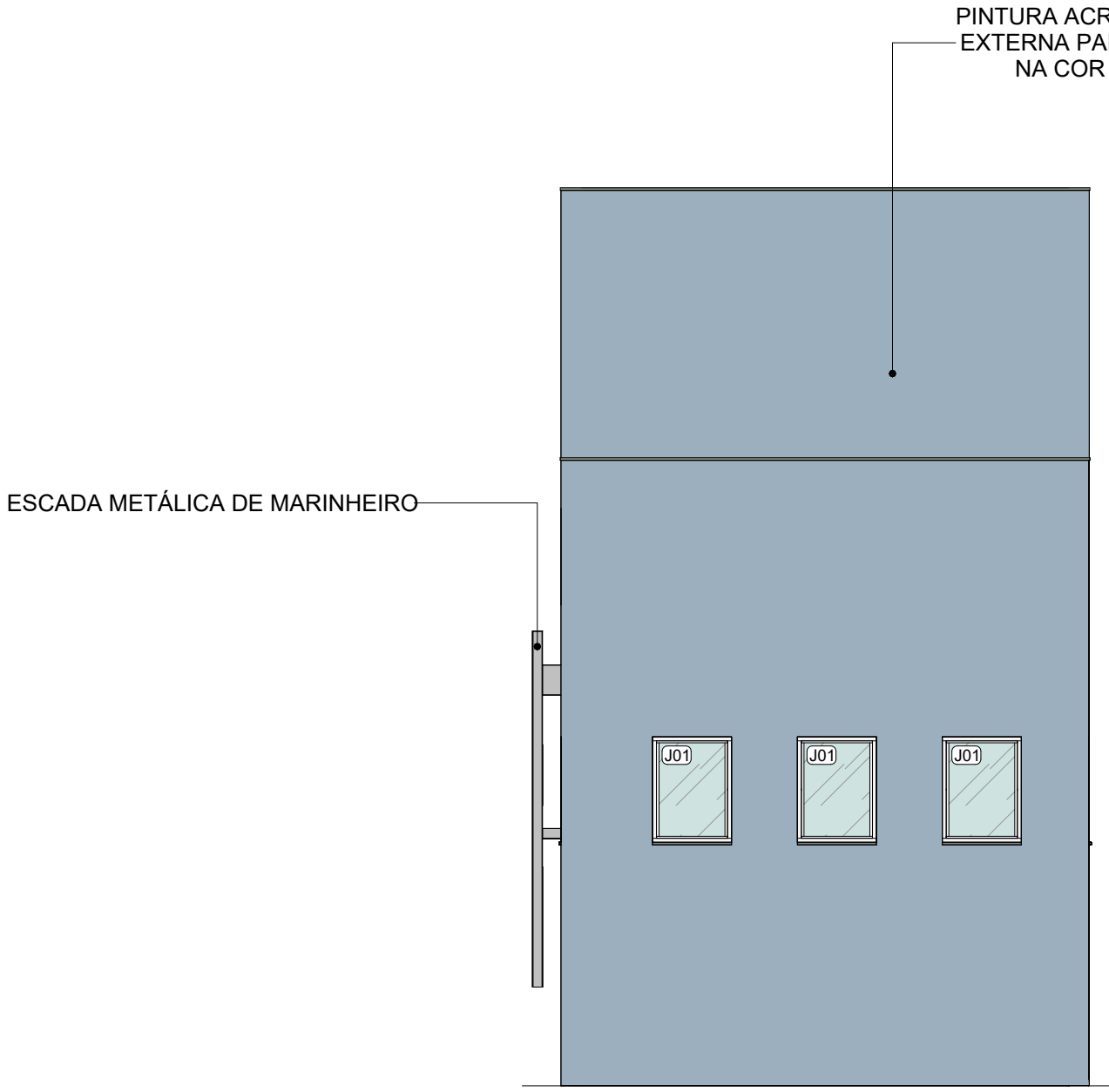
3 FACHADA LATERAL ESQUERDA - VESTIÁRIO ESCALA: 1 : 50
