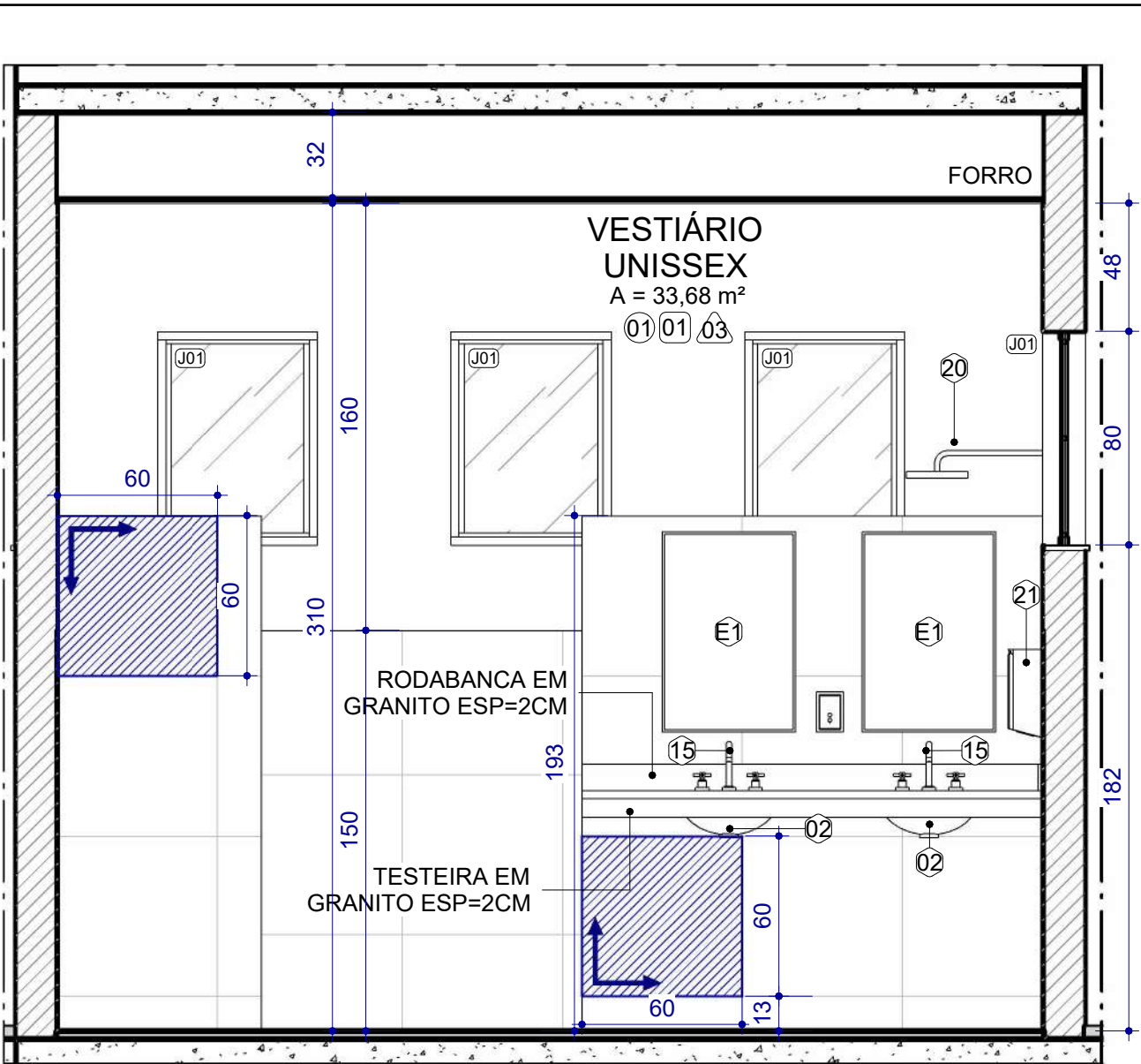
B REFORMA - ELEVAÇÃO D - VESTIÁRIO UNISSEX ESCALA: 1 : 25
