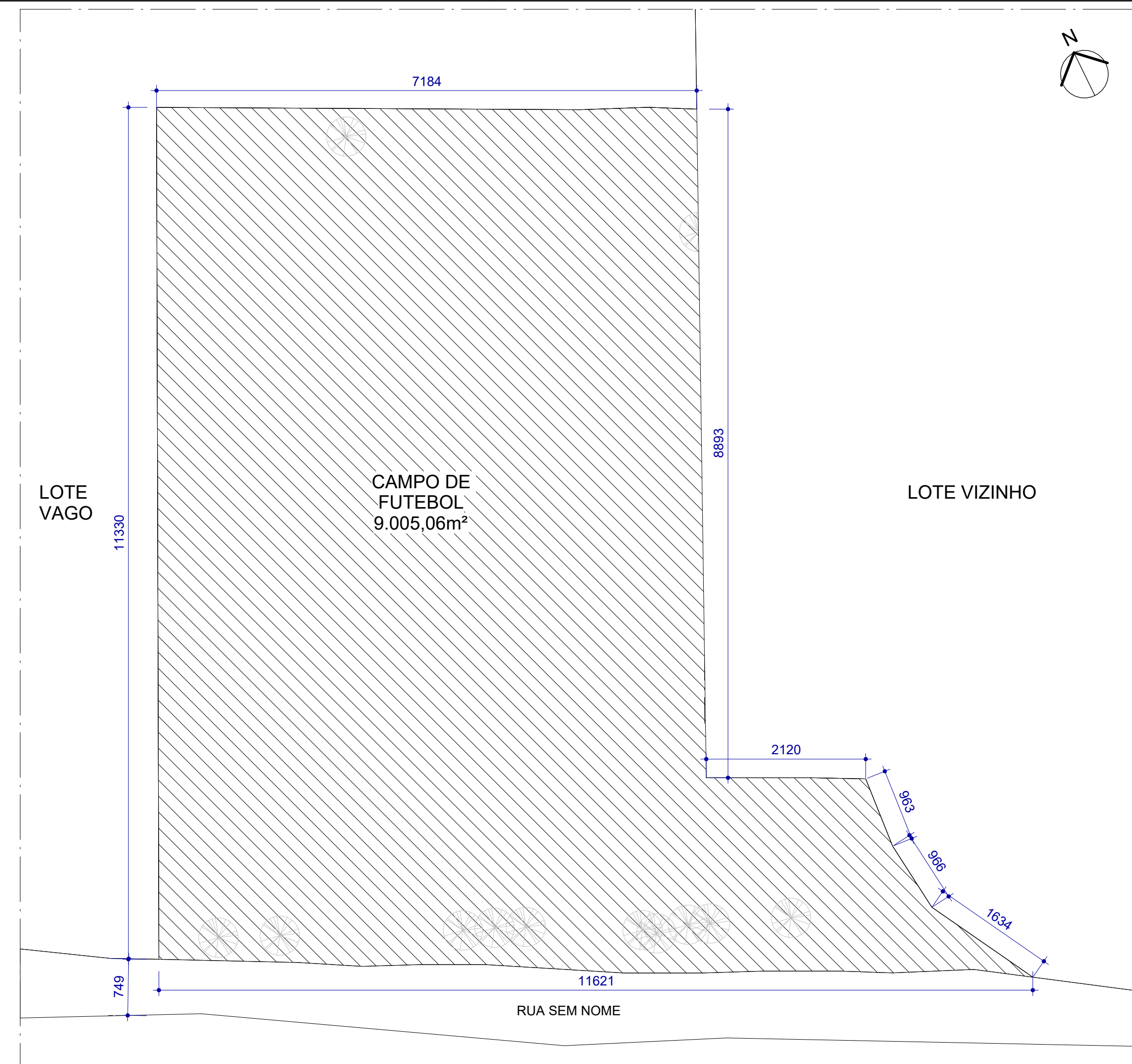
2 PLANTA DE SITUAÇÃO ESCALA: 1 : 500
