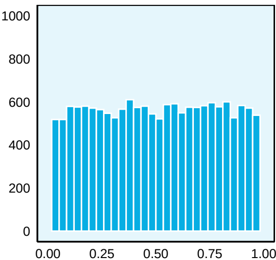
Edge_ORA
