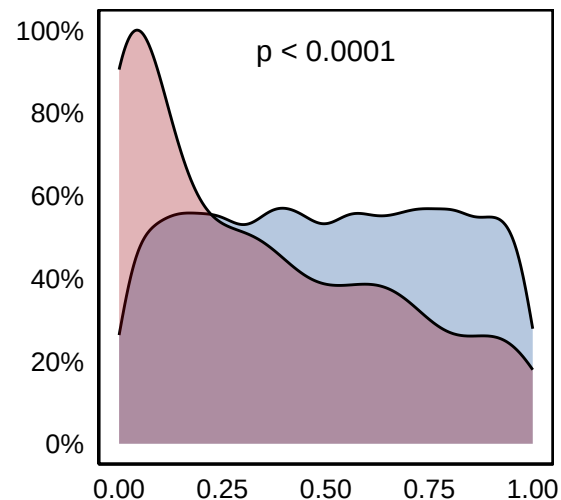
Edge_ORA
