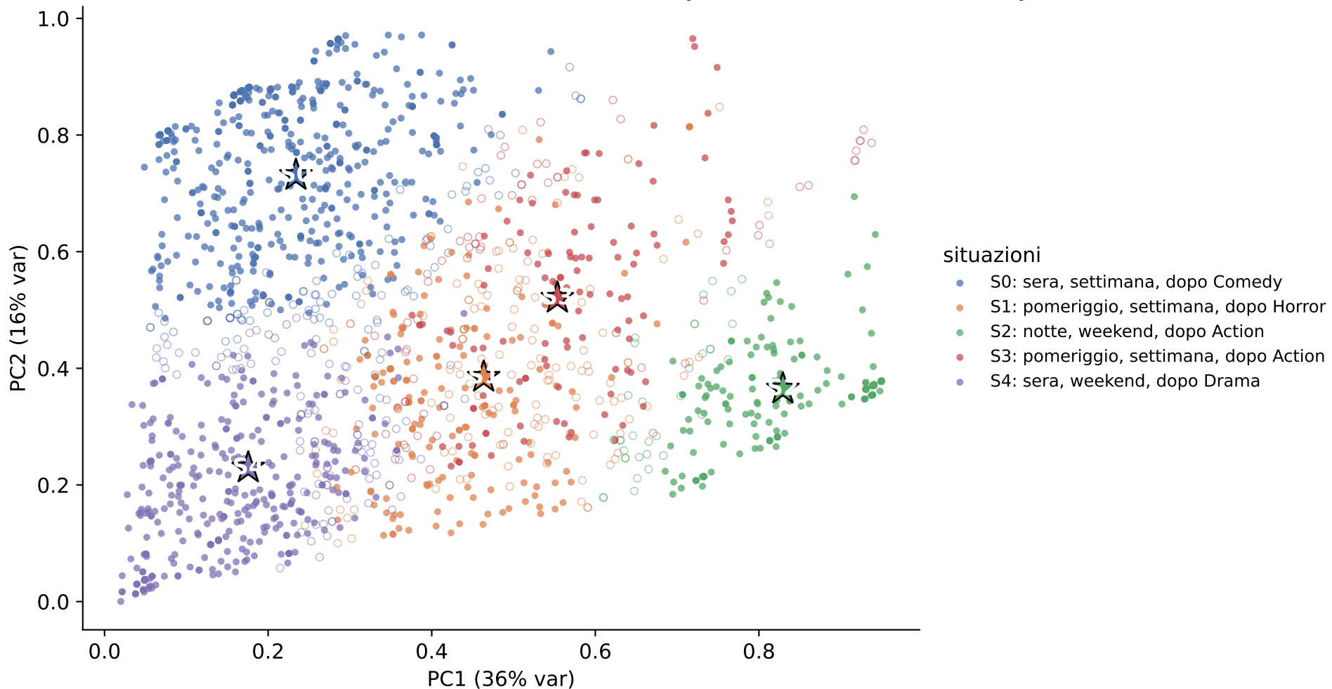
Spazio delle situazioni — ml1m (★=centroide, ○=boundary/incertezza, 24% boundary)
