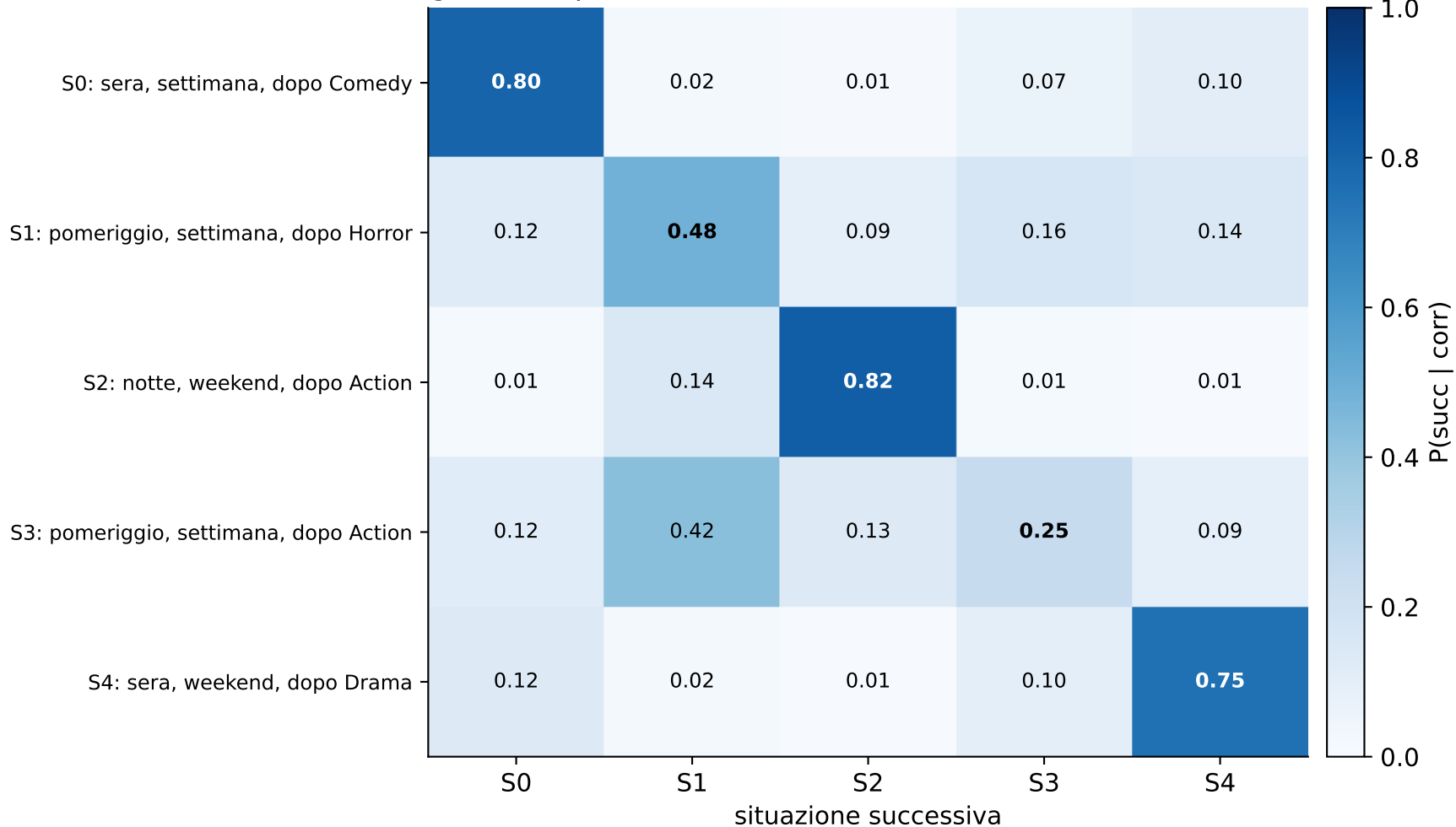
Proiezione L3 — dove si muove la situazione (Markov) — ml1m diagonale = persistenza (es. S2 stabile 82%, S3 transitoria 25%)
