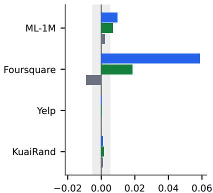
AFM
