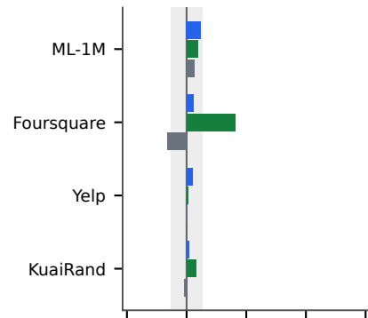
DeepFM
