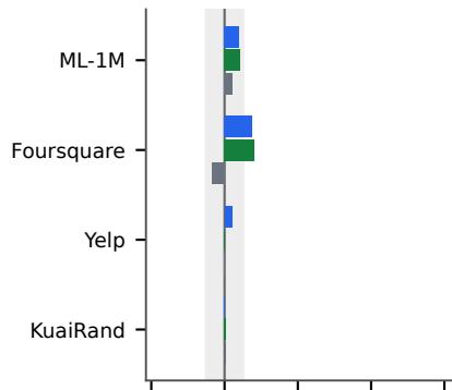
FPMC
