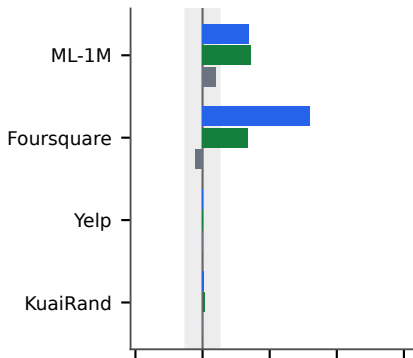
AFM
