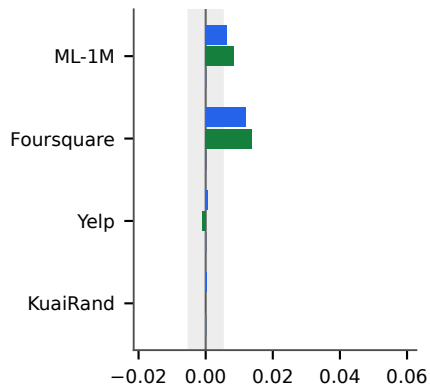
FPMC
