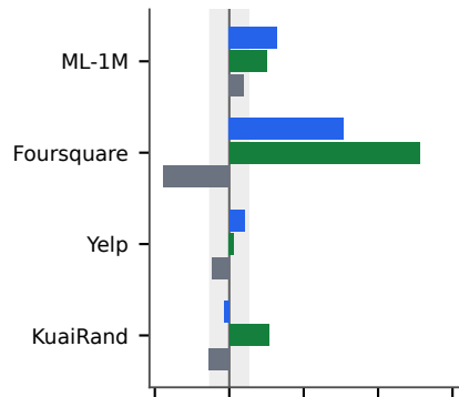
SASRec
