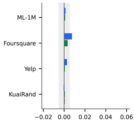
SASRec
