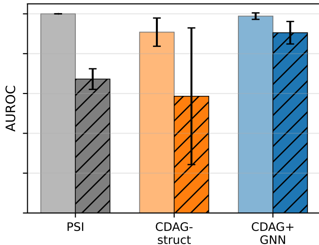
AUROC
