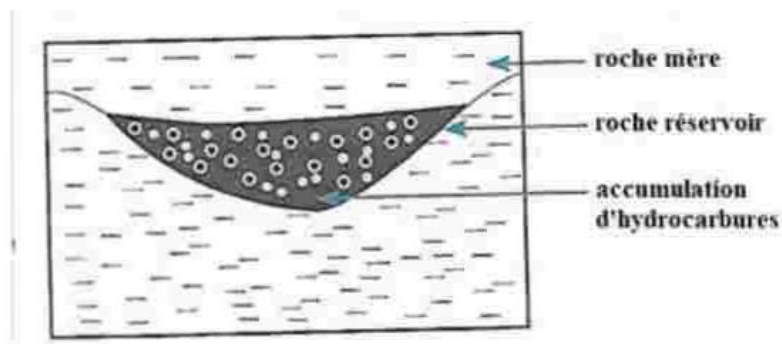
PIÈGE STRATIGRAPHIQUE
