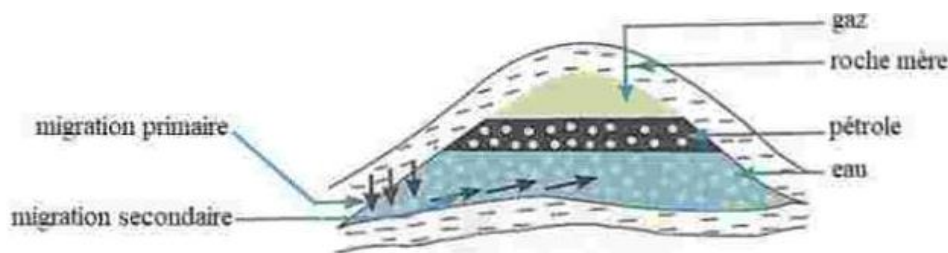
PIÈGE STRUCTURAL
