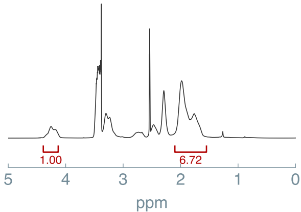
^1\text{H} NMR
