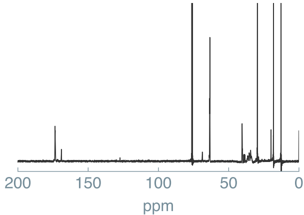
^{13}\text{C} NMR
