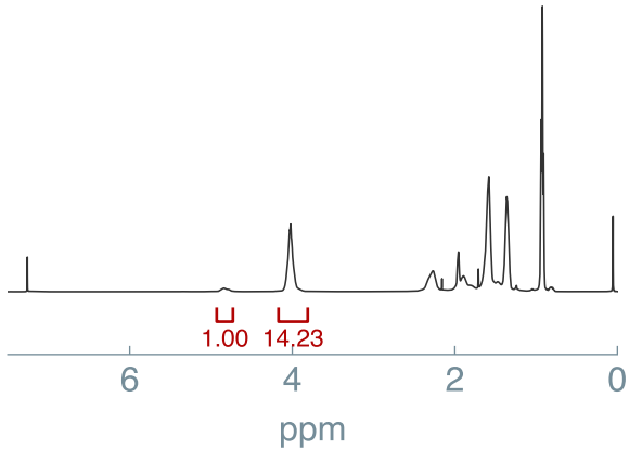
^1\text{H} NMR
