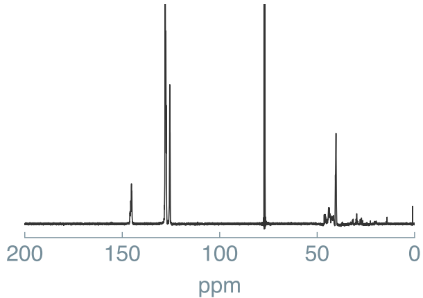
^{13}\text{C} NMR
