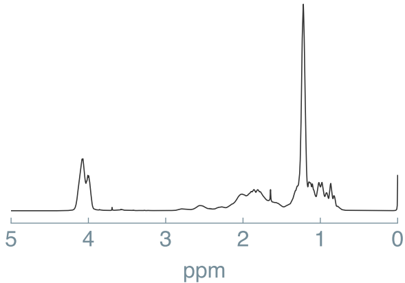
^1\text{H} NMR
