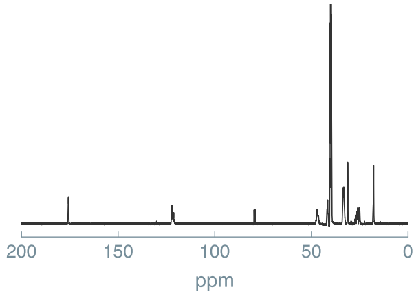
^{13}\text{C} NMR
