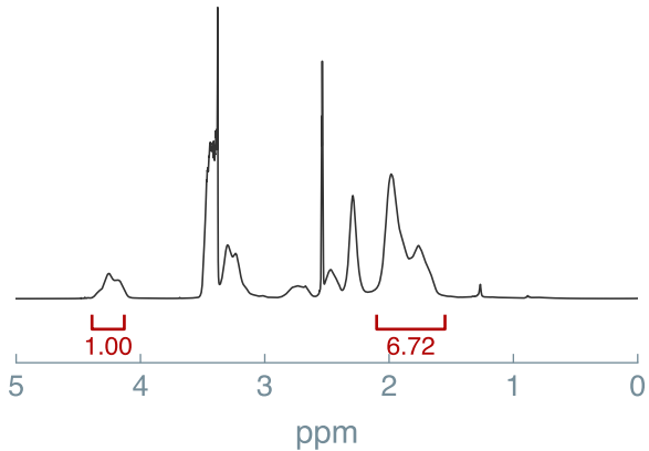
^1\text{H} NMR
