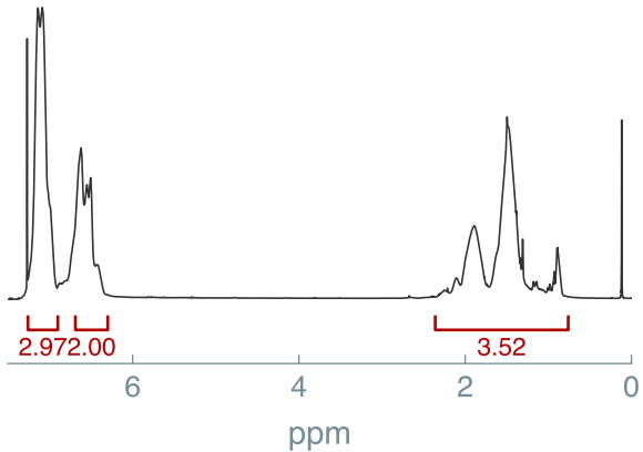
^1\text{H} NMR
