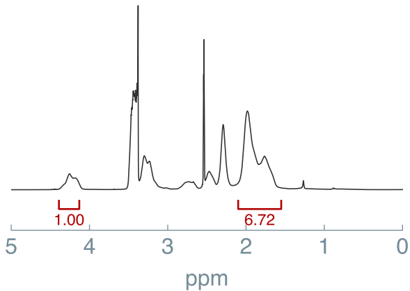
^1\text{H} NMR
