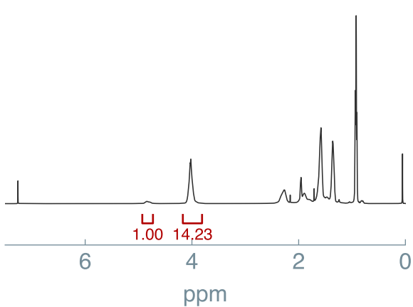
^1\text{H} NMR
