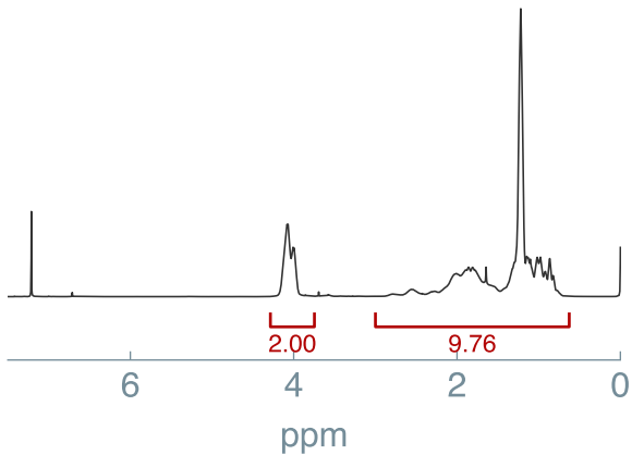
^1\text{H} NMR
