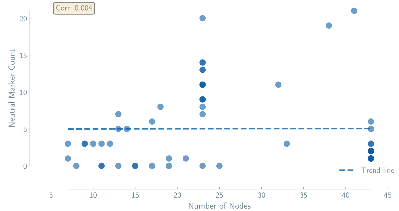
ToolCallingAgent + gpt-4o (n=60)
