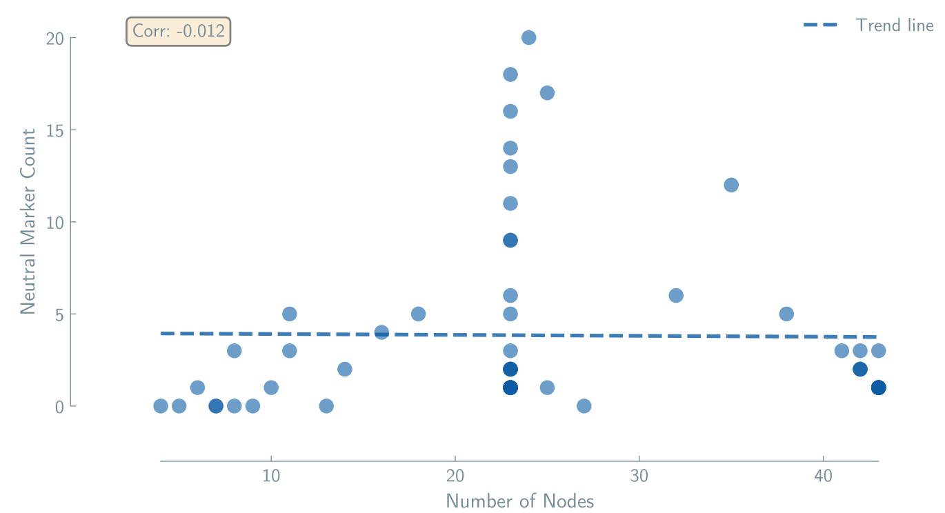
ToolCallingAgent + gpt-4o (n=60)
