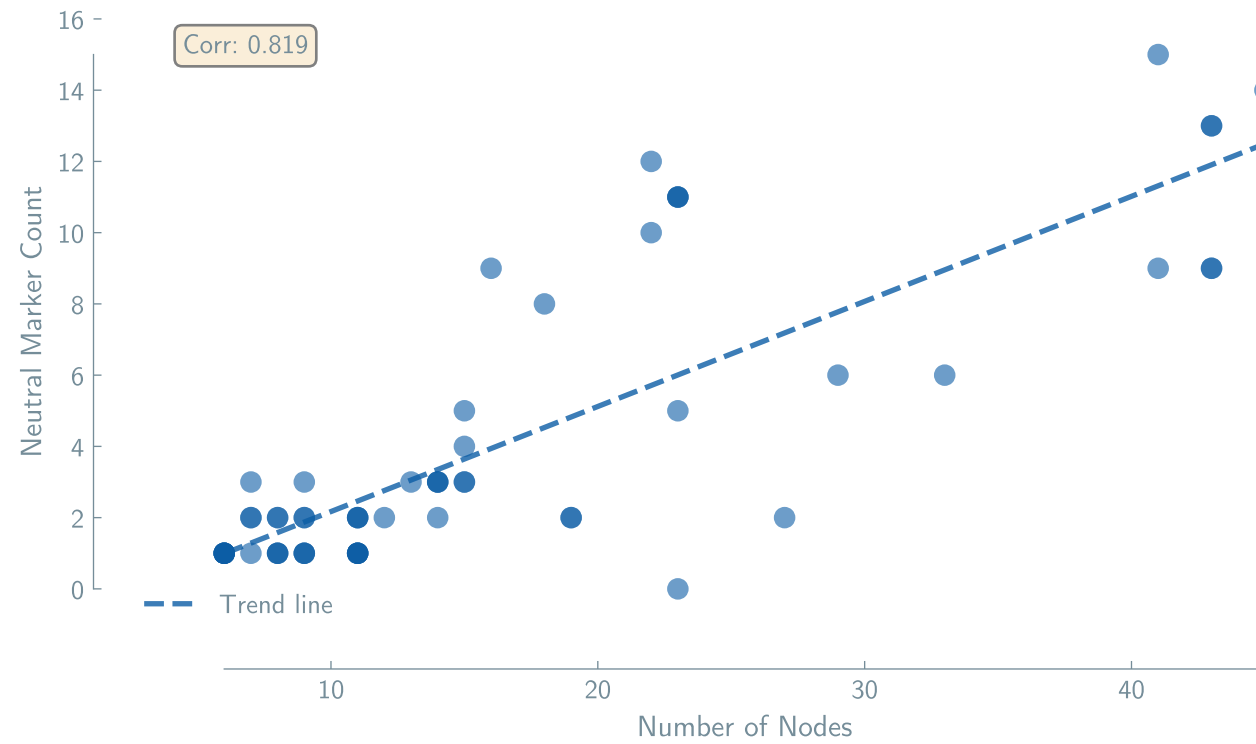
ToolCallingAgent + claude_sonnet_45 (n=60)
