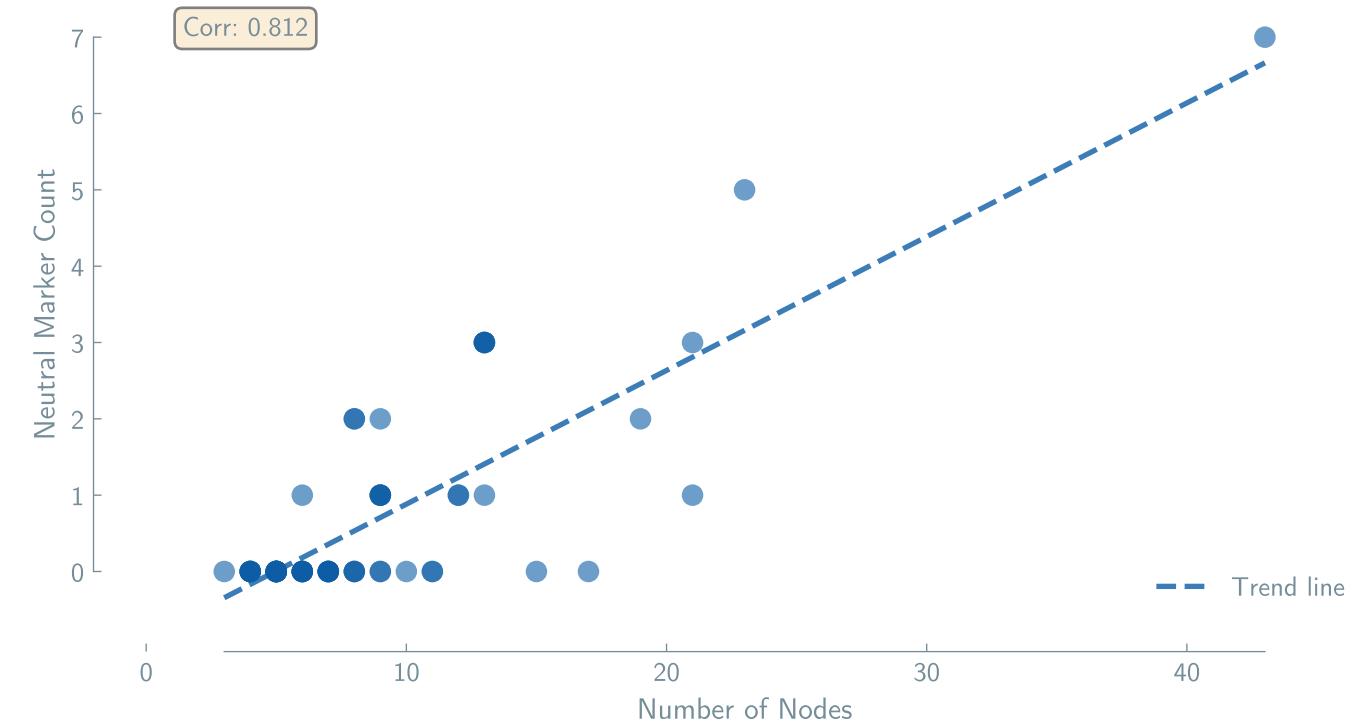
ToolCallingAgent + claude_sonnet_45 (n=60)
