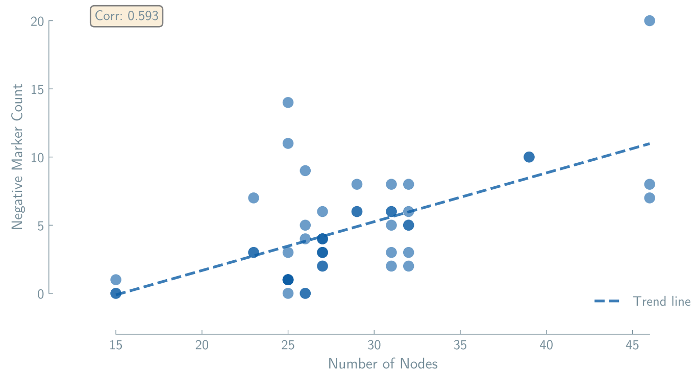
ToolCallingAgent + gpt-4o (n=49)
