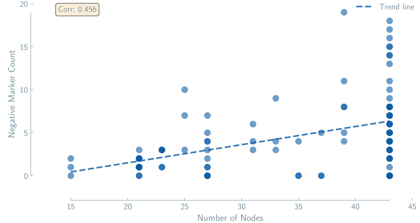
ToolCallingAgent + gpt-4o (n=112)
