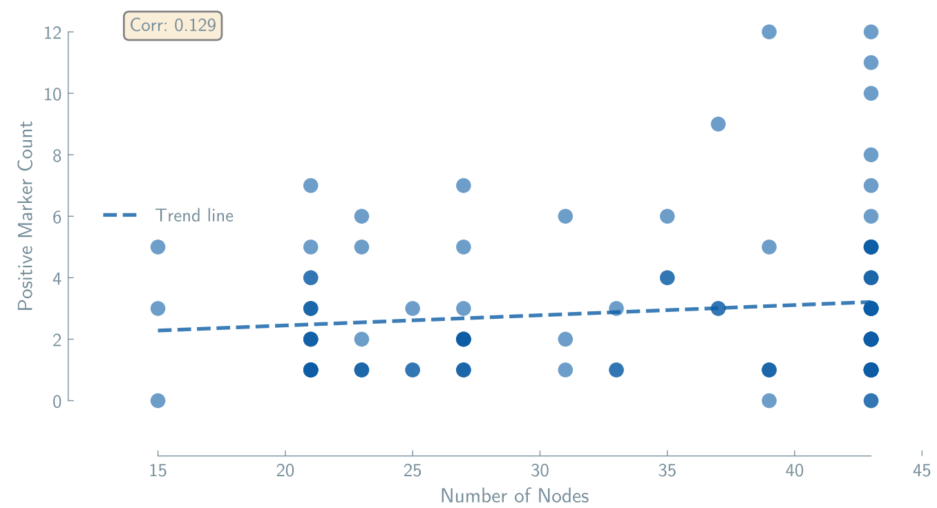
ToolCallingAgent + gpt-4o (n=112)
