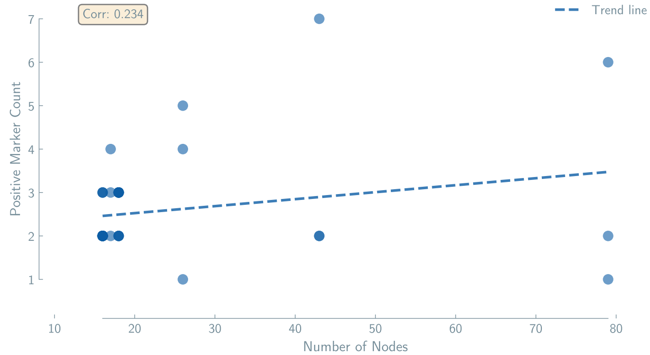
ToolCallingAgent + claude_sonnet_45 (n=45)
