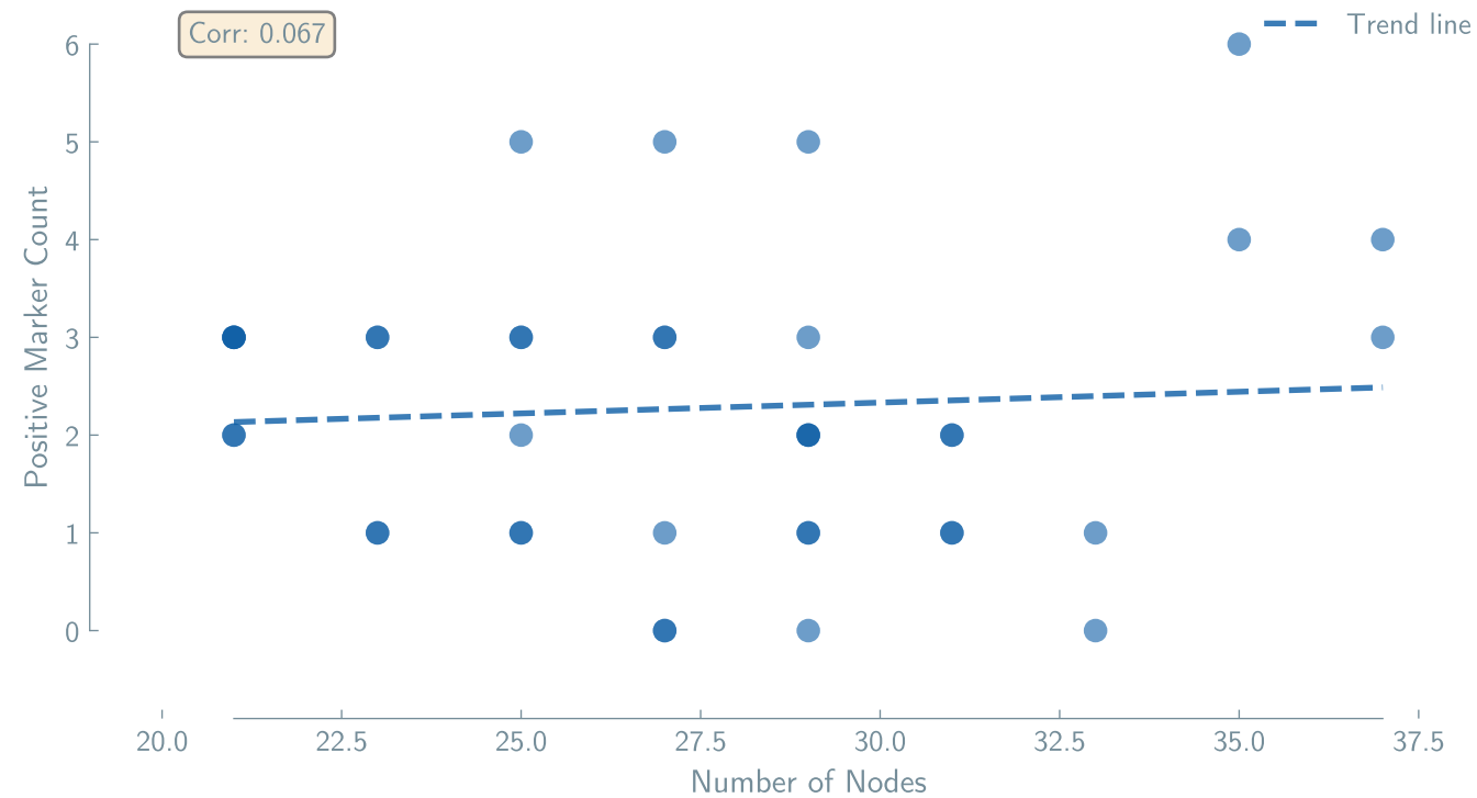
ToolCallingAgent + gpt-4o (n=36)
