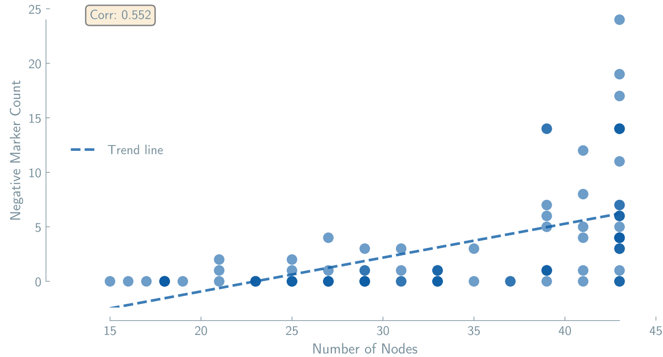
ToolCallingAgent + claude_sonnet_45 (n=95)
