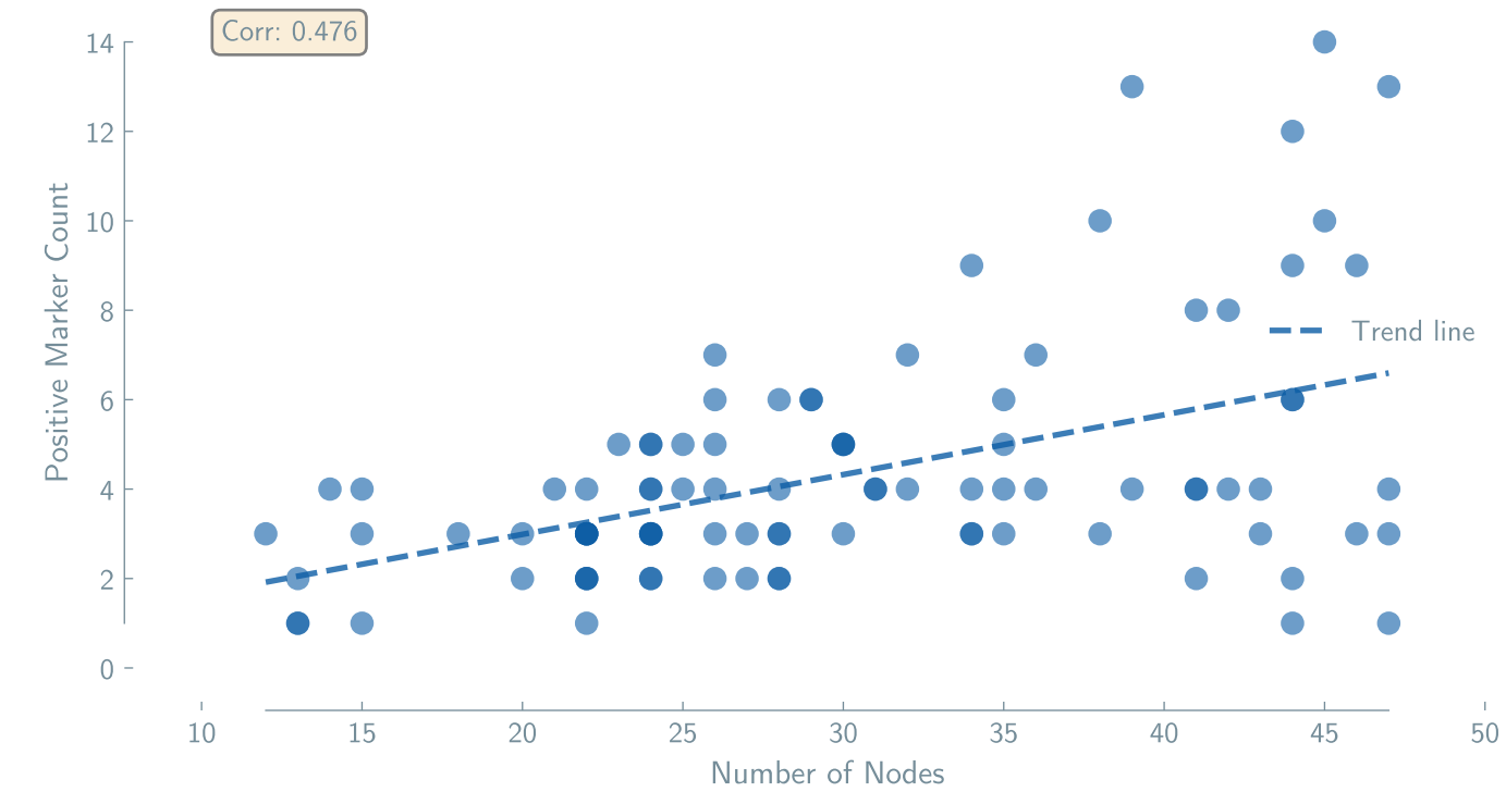
ToolCallingAgent + claude_sonnet_45 (n=95)
