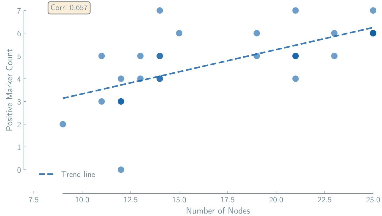
ToolCallingAgent + claude_sonnet_45 (n=30)
