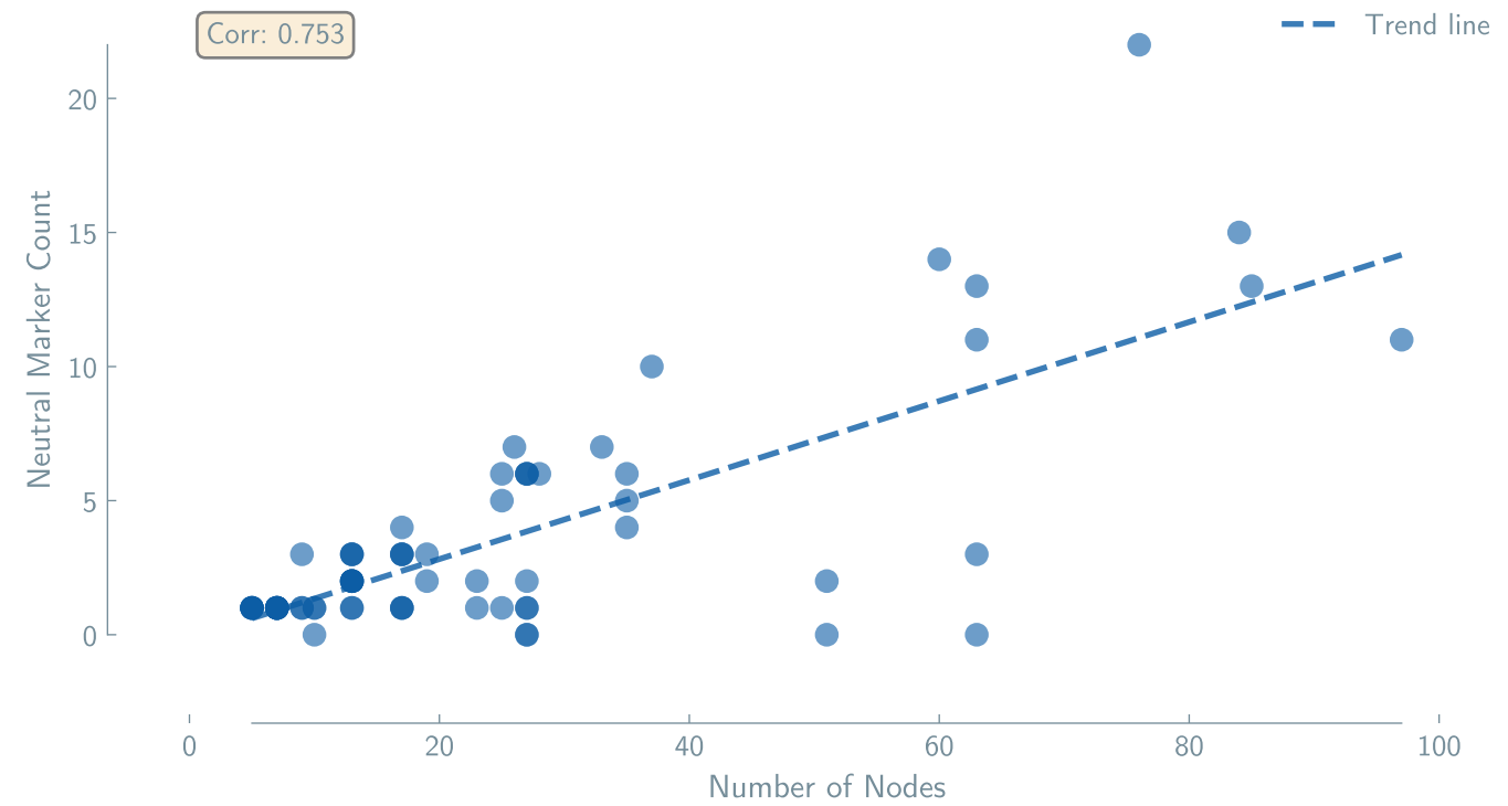
ToolCallingAgent + gpt-4o (n=72)
