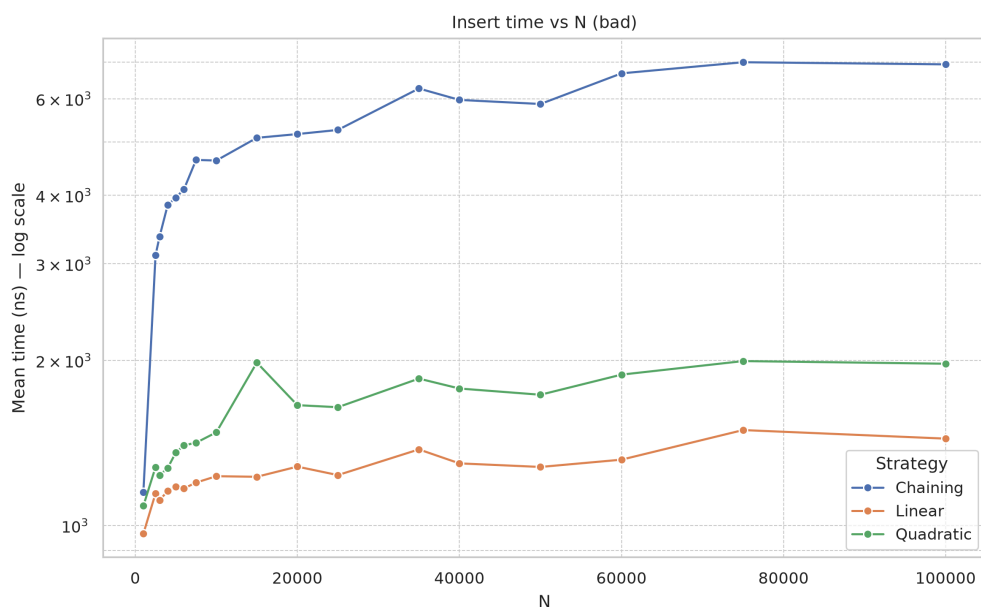
Рисунок 8. Время вставки (ключи с коллизиями)
