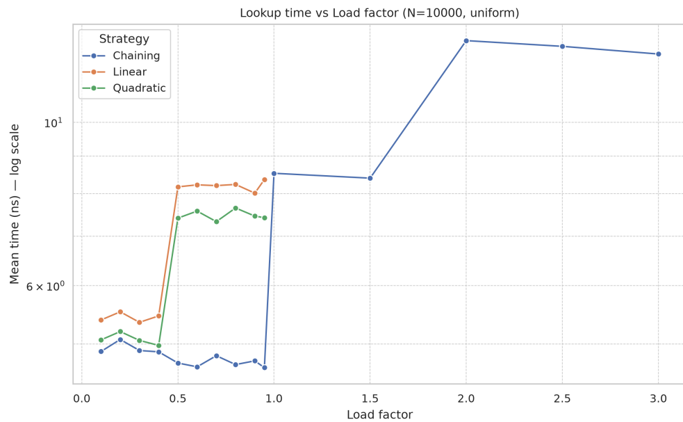
Рисунок 13. Время поиска от load factor (равномерные ключи, N=10000)
