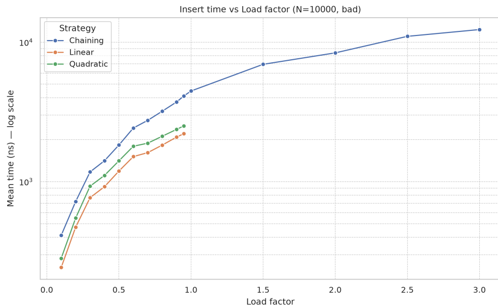
Рисунок 14. Время вставки от load factor (плохие ключи, N=10000)
