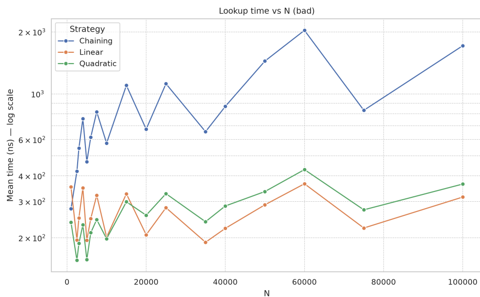
Рисунок 9. Время поиска (ключи с коллизиями)
