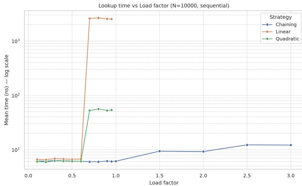
Рисунок 11. Время поиска от load factor (последовательные ключи, N=10000)
