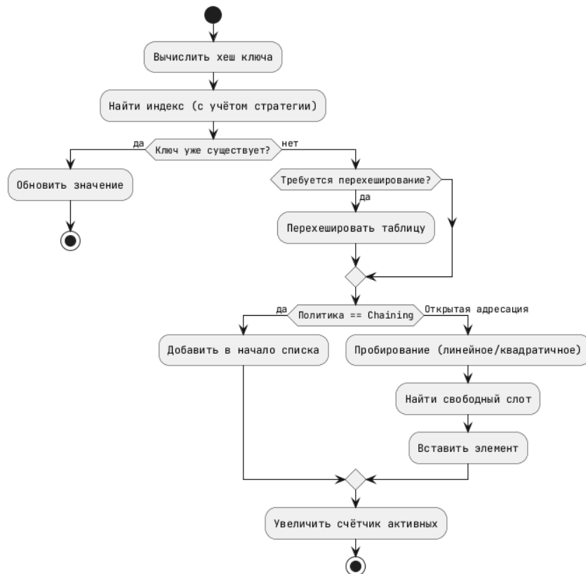
Рисунок 2. Алгоритм вставки элемента
