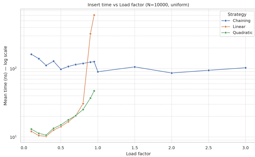
Рисунок 12. Время вставки от load factor (равномерные ключи, N=10000)
