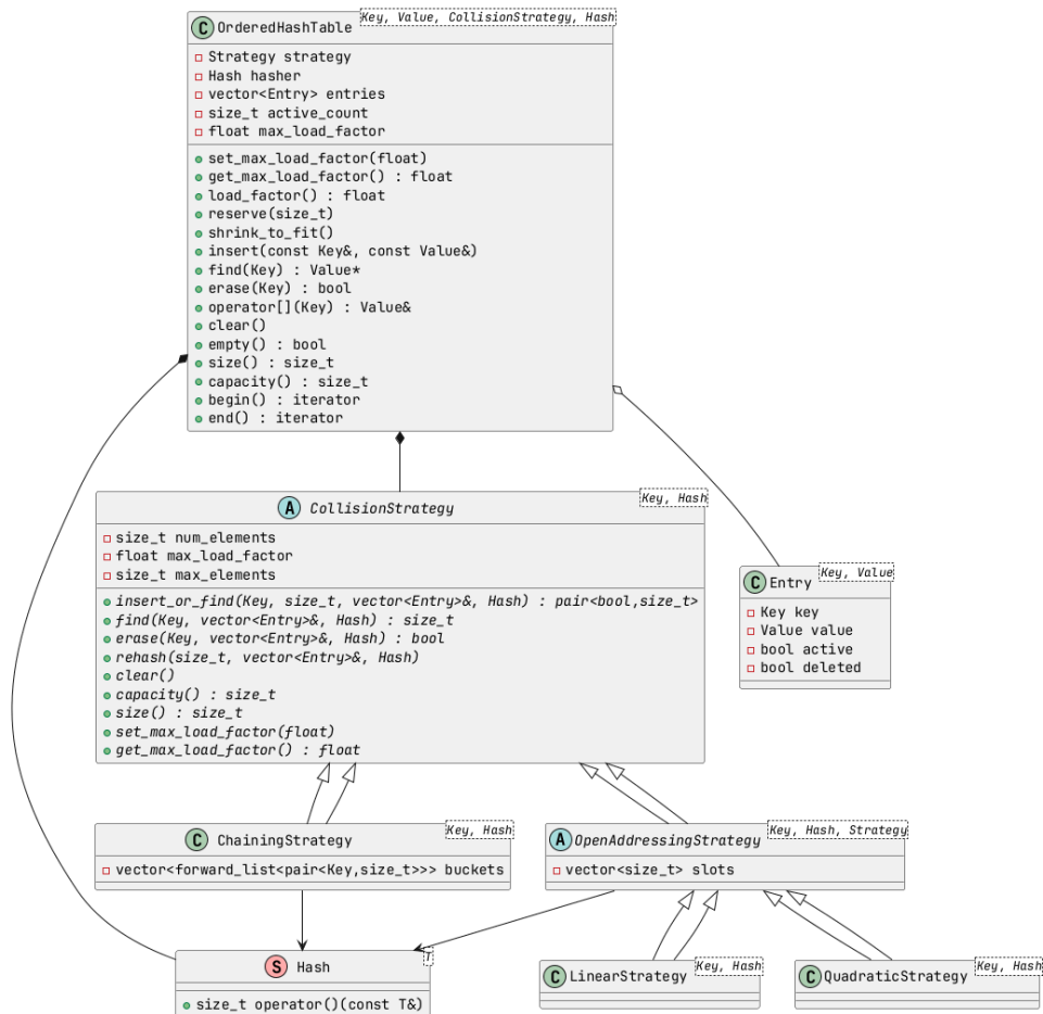
Рисунок 1. UML-диаграмма классов
