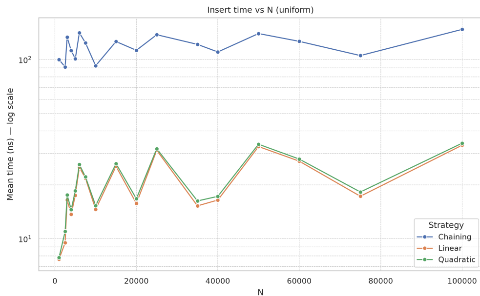
Рисунок 6. Время вставки (равномерные ключи)
