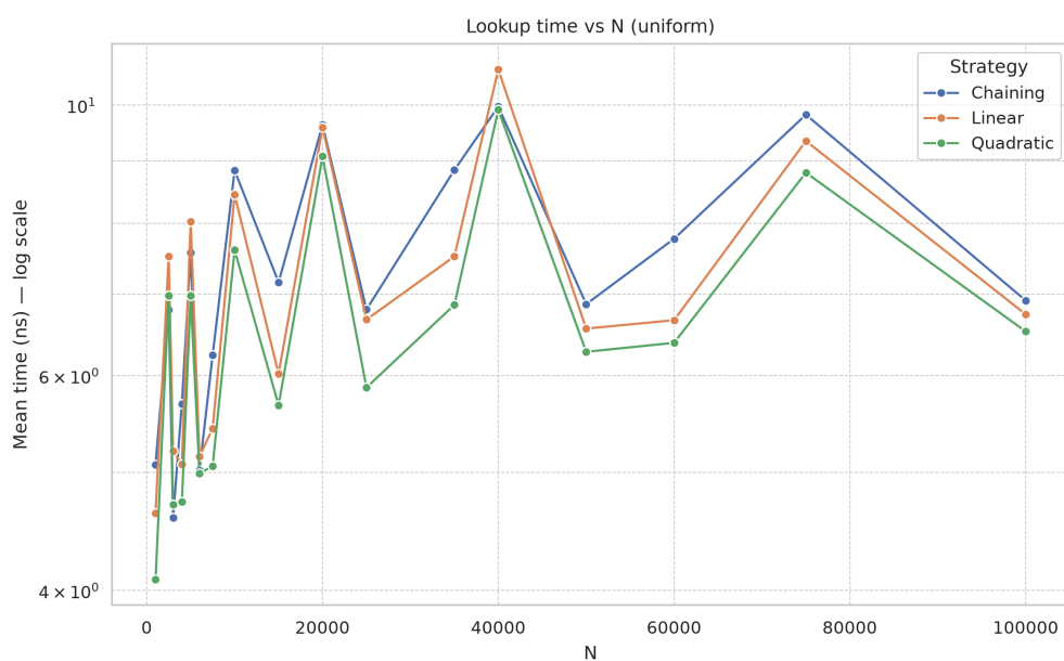
Рисунок 7. Время поиска (равномерные ключи)
