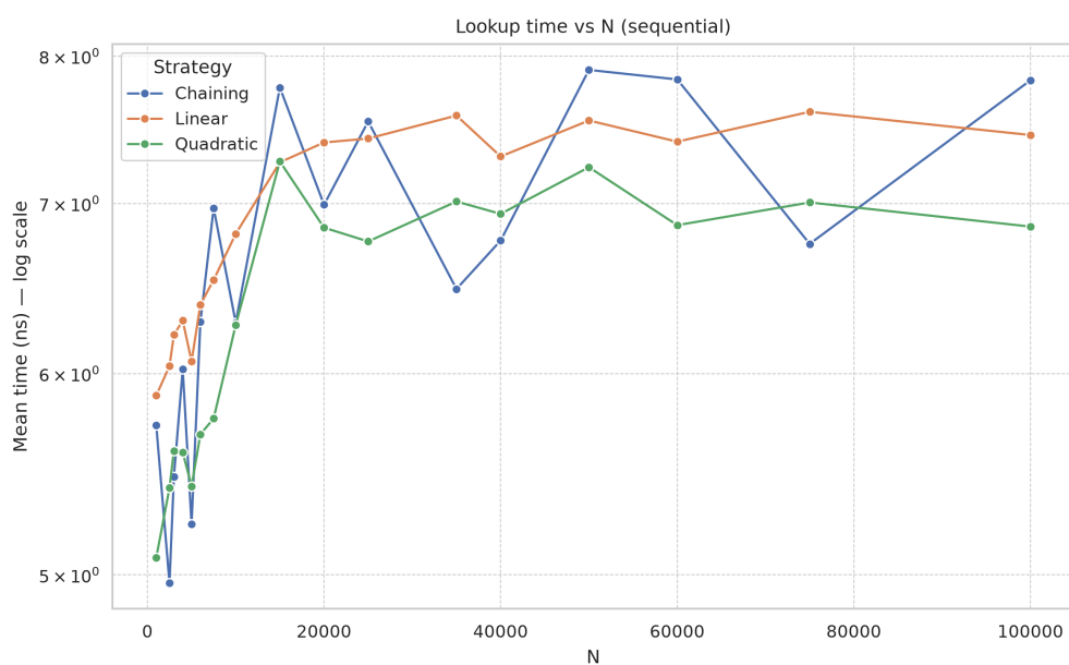
Рисунок 5. Время поиска (последовательные ключи)
