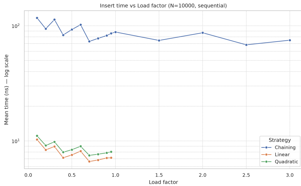
Рисунок 10. Время вставки от load factor (последовательные ключи, N=10000)
