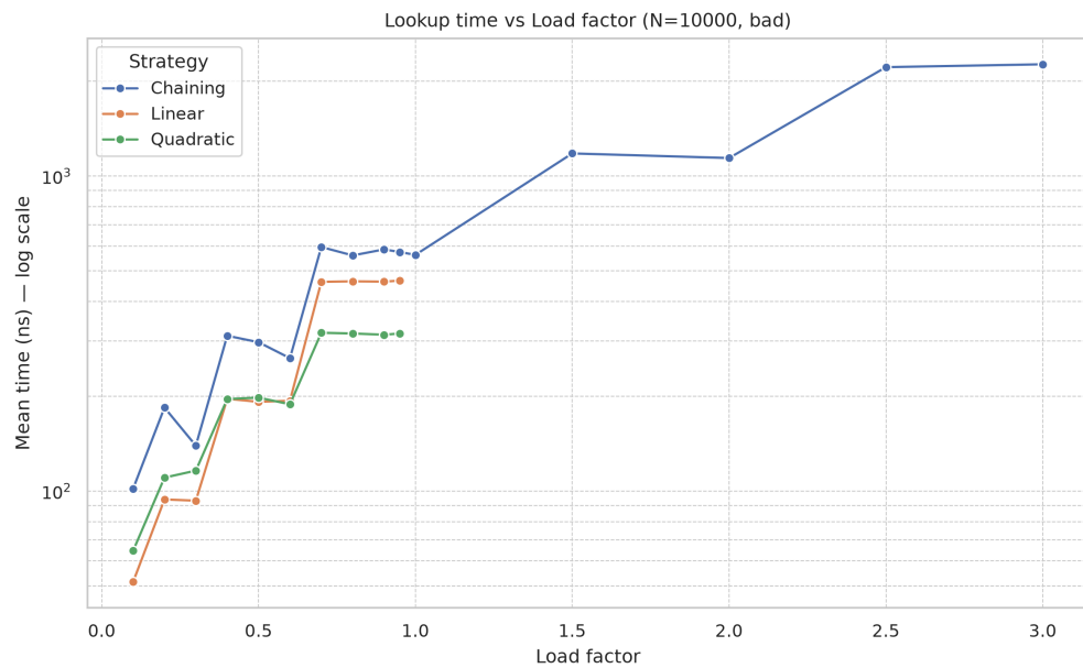
Рисунок 15. Время поиска от load factor (плохие ключи, N=10000)
