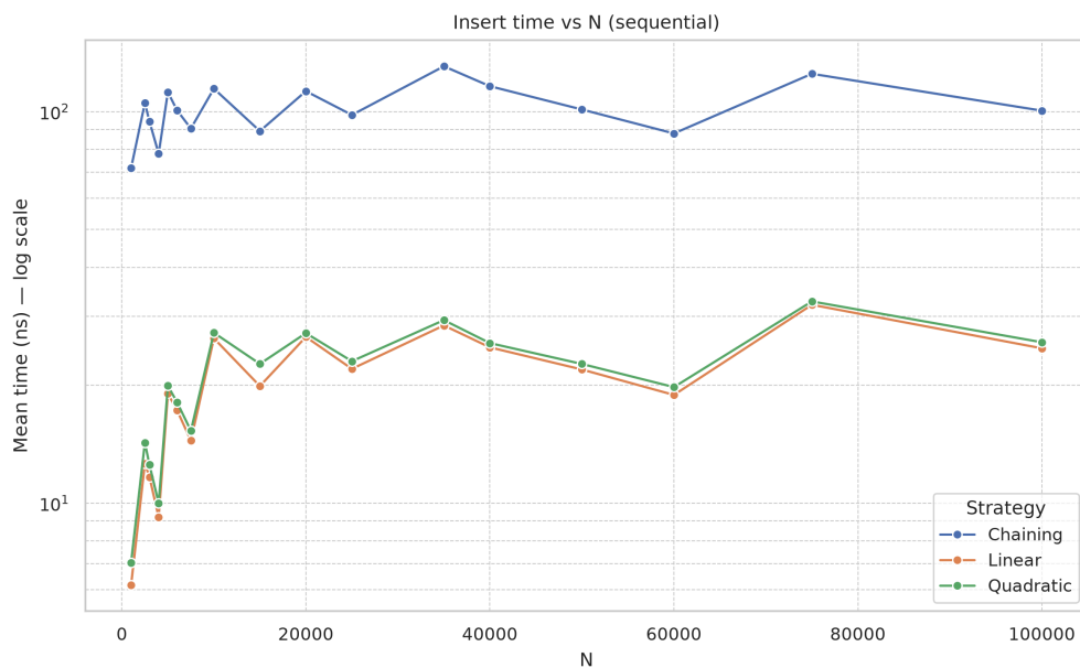
Рисунок 4. Время вставки (последовательные ключи)
