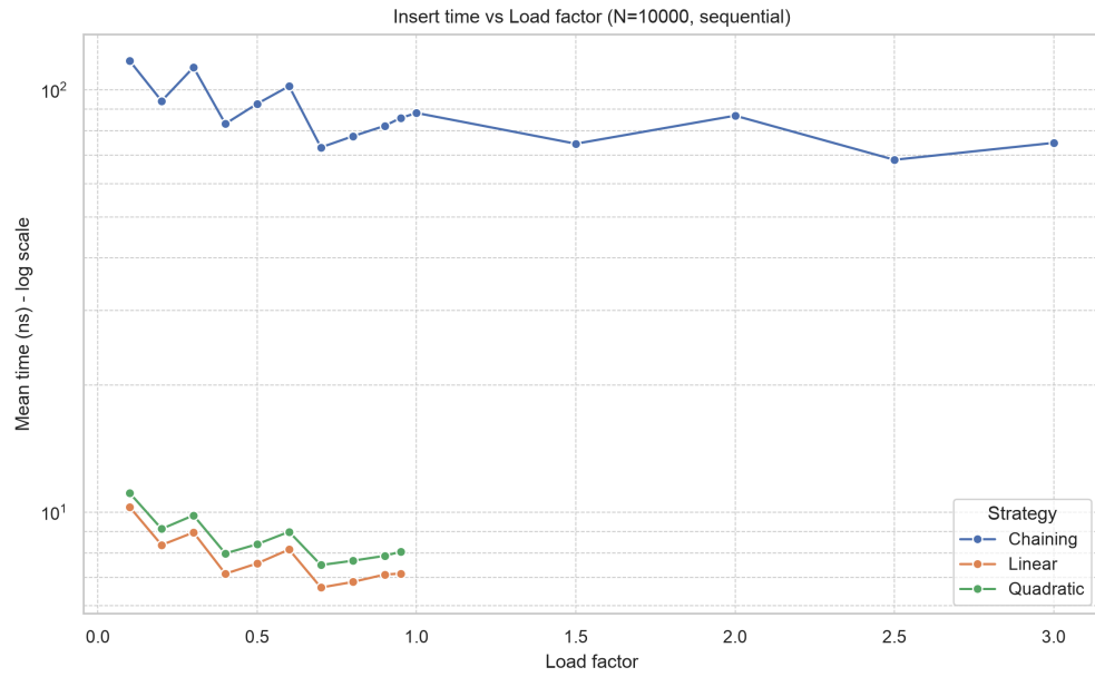
Рисунок 13. Время вставки от load factor (последовательные ключи, N=10000)
