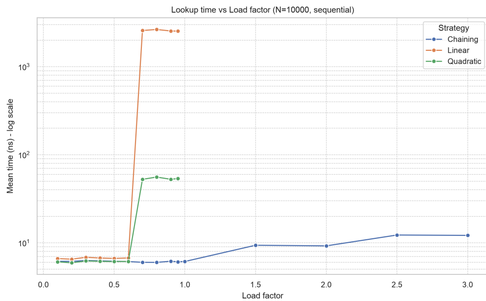
Рисунок 14. Время поиска от load factor (последовательные ключи, N=10000)
