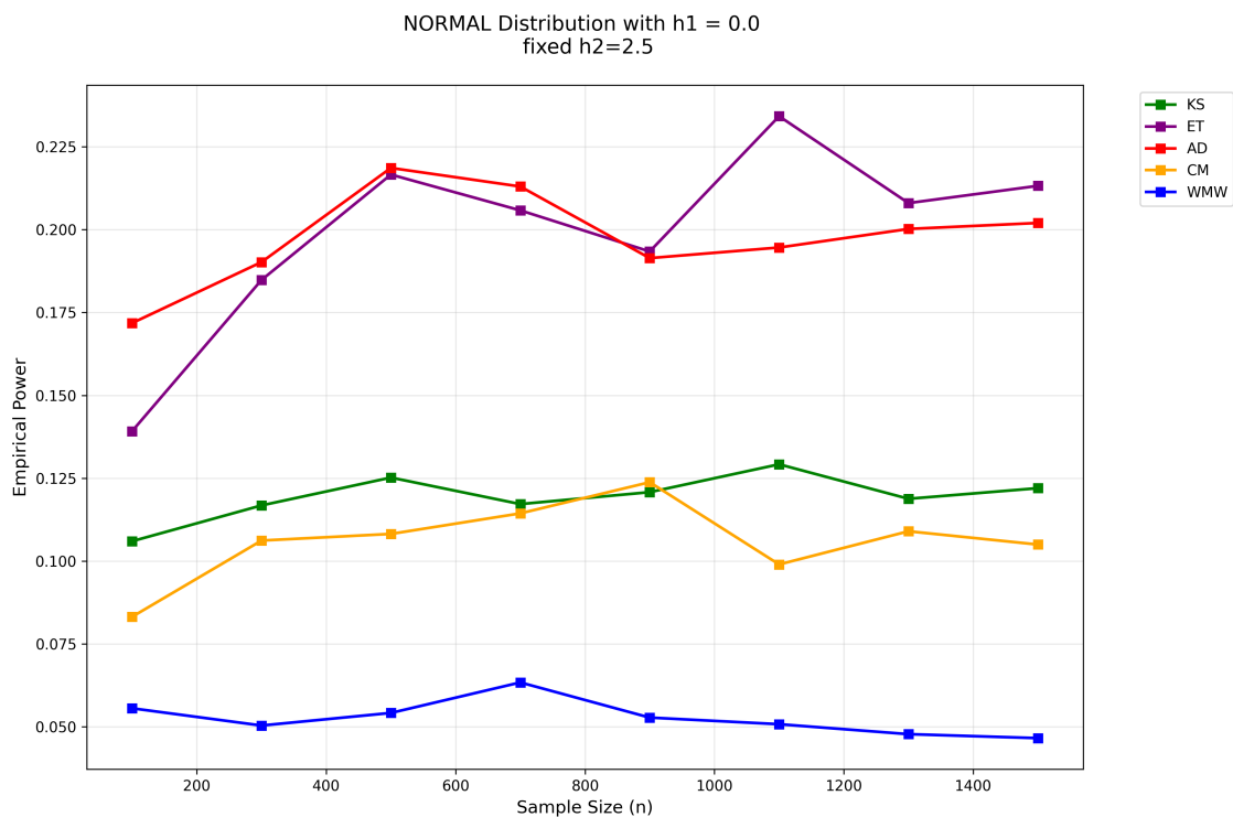
Рис. 9: Зависимость эмпирических мощностей от размера выборки в случае стандартных нормальных распределений, отличающихся масштабом.
