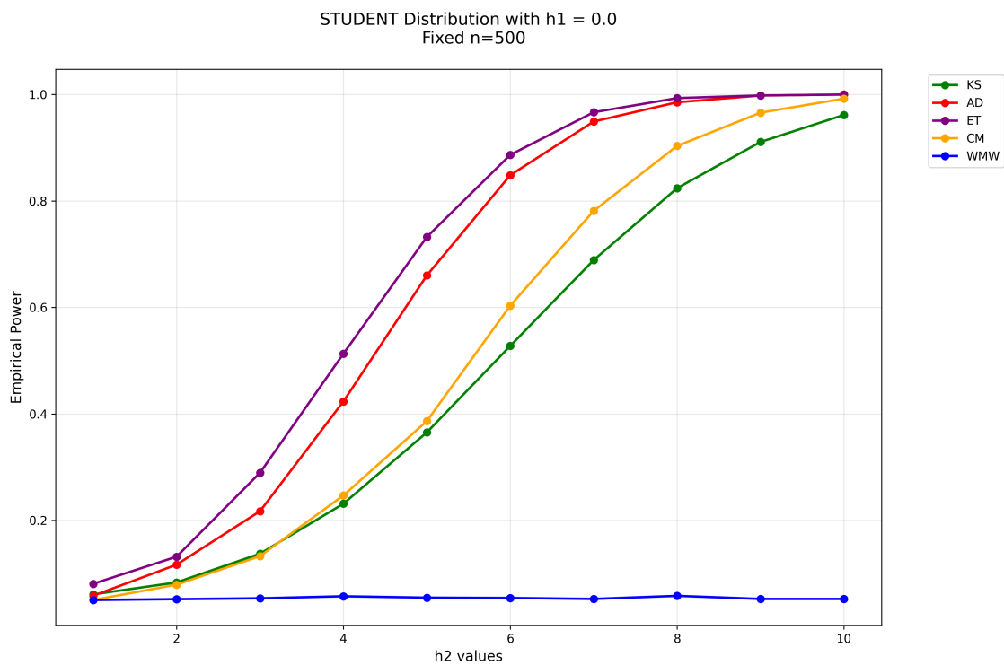
Рис. 7: Зависимость эмпирических мощностей от различия по сдвигу, в случае распределений Стьюдента ( df=20 ) с одинаковым масштабом.
