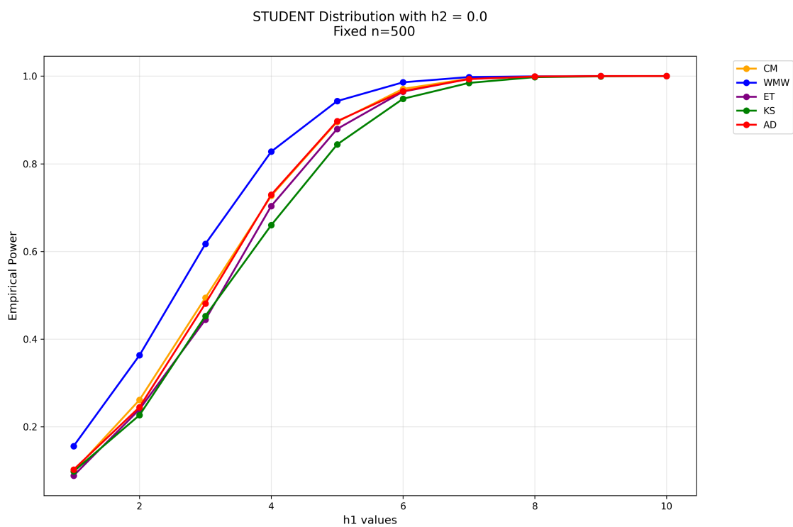
Рис. 6: Зависимость эмпирических мощностей от различия по сдвигу, в случае распределений Стьюдента ( df=10 ) с одинаковым масштабом.
