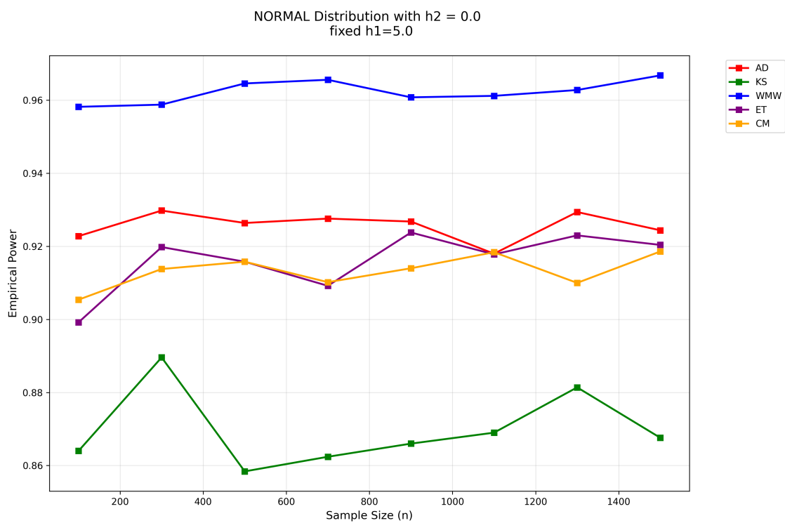
Рис. 10: Зависимость эмпирических мощностей от размера выборки в случае стандартных нормальных распределений, отличающихся сдвигом.
