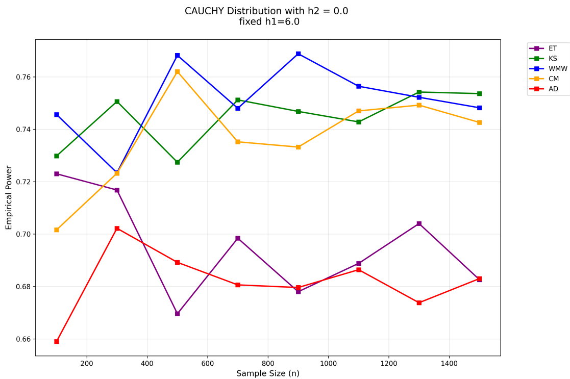
Рис. 12: Зависимость эмпирических мощностей от размера выборки в случае стандартных распределений Коши, отличающихся сдвигом.
