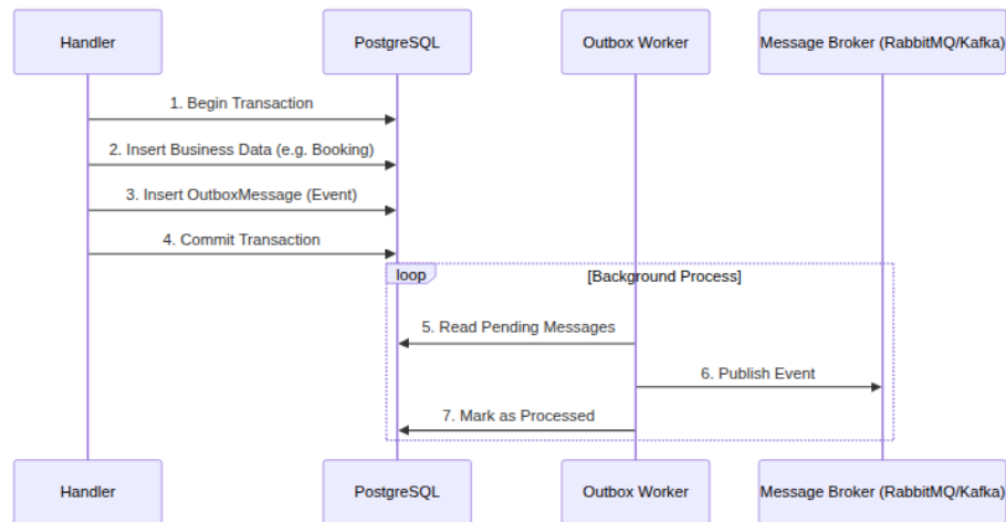
Hình 2.8. Sơ đồ Tuần tự (Sequence Diagram) cơ chế Transactional Outbox
