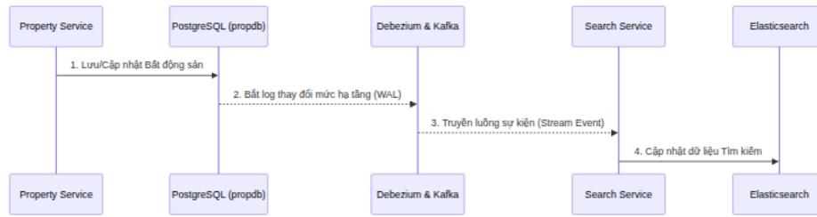
Hình 2.3. Sơ đồ Tuần tự minh họa giao tiếp Đồng bộ dữ liệu qua Kafka
