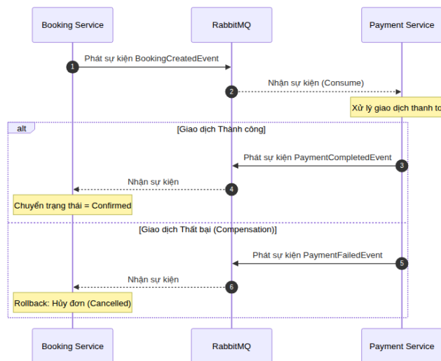
Hình 2.4. Sơ đồ Tuần tự minh họa giao tiếp Đặt phòng qua RabbitMQ
