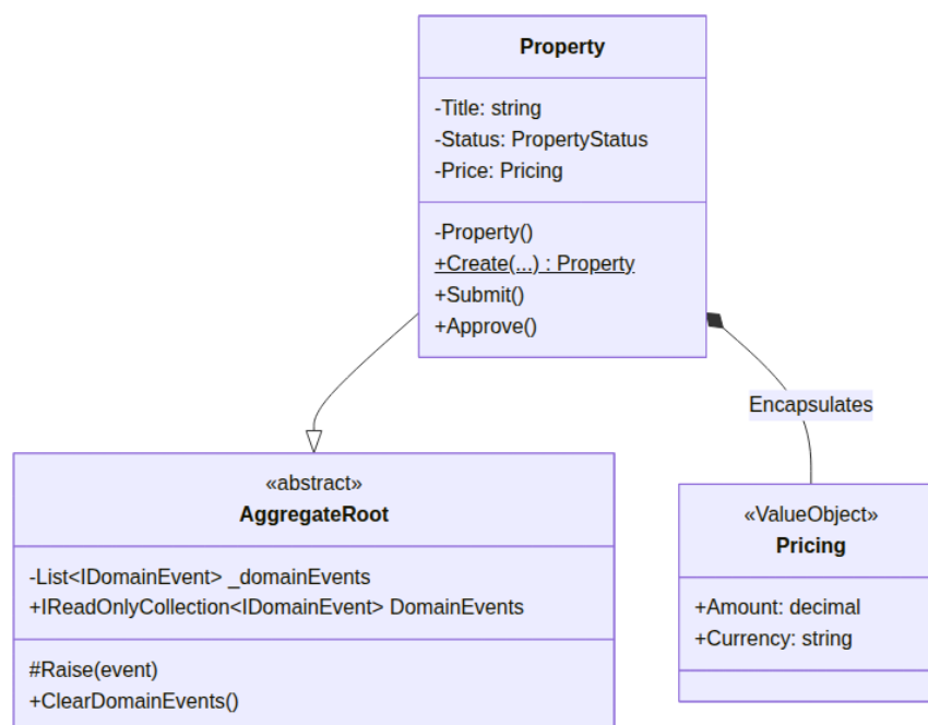
Hình 2.11. Sơ đồ Lớp (Class Diagram) mô tả Aggregate Root trong DDD
