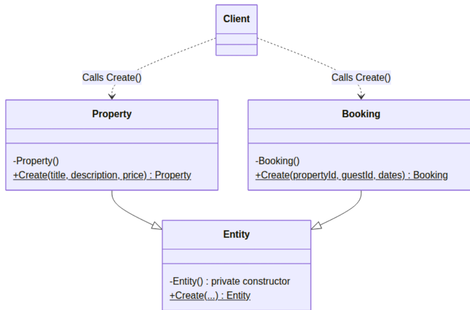
Hình 2.12. Sơ đồ Lớp (Class Diagram) của Factory Method Pattern
