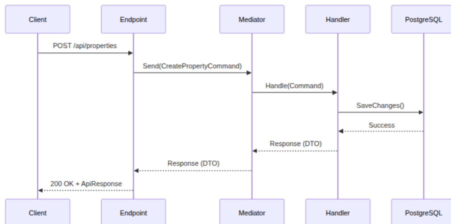
Hình 2.7. Sơ đồ Tuần tự (Sequence Diagram) minh họa luồng xử lý CQRS
