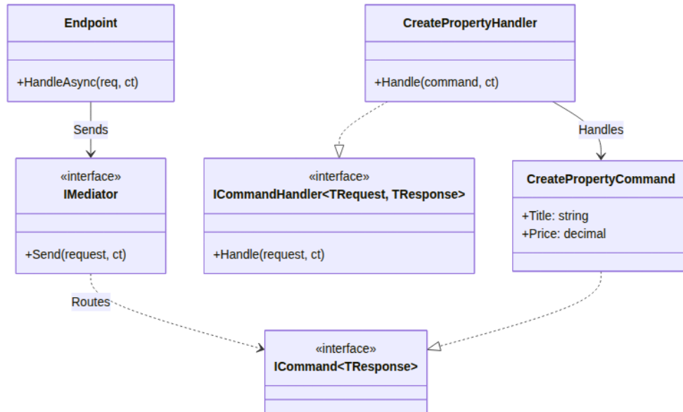
Hình 2.6. Sơ đồ Lớp (Class Diagram) cấu trúc CQRS sử dụng Mediator
