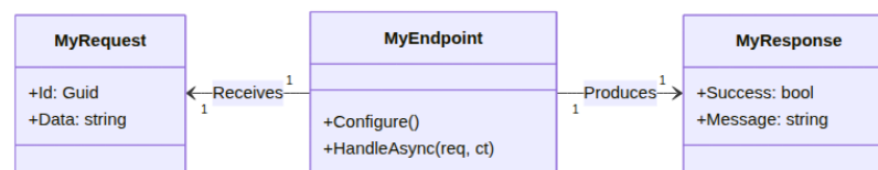
Hình 2.5. Sơ đồ Lớp (Class Diagram) cấu trúc REPR Pattern
