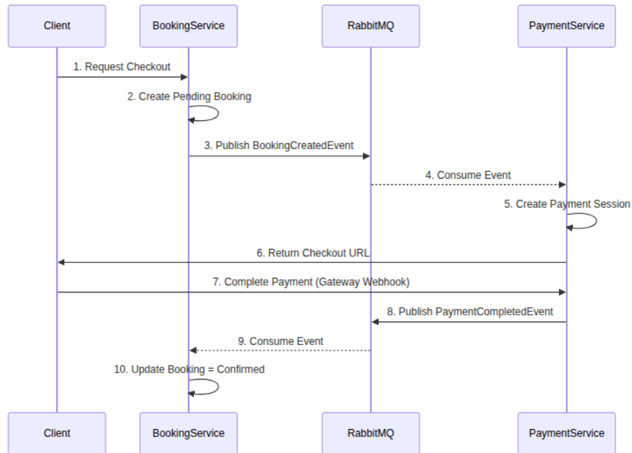
Hình 2.9. Sơ đồ Tuần tự (Sequence Diagram) minh họa Saga Pattern giữa Booking và Payment
