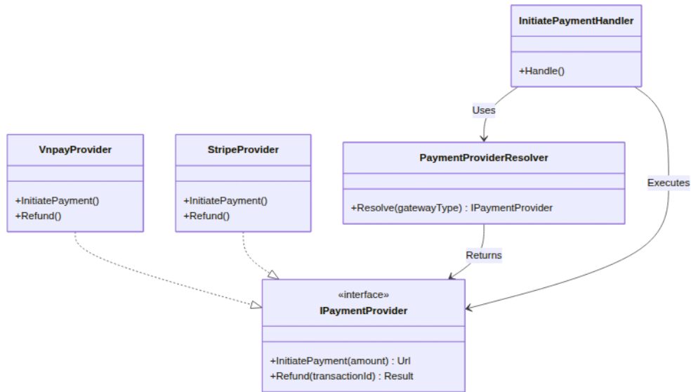
Hình 2.10. Sơ đồ Lớp (Class Diagram) mô hình Strategy Pattern tại PaymentService
