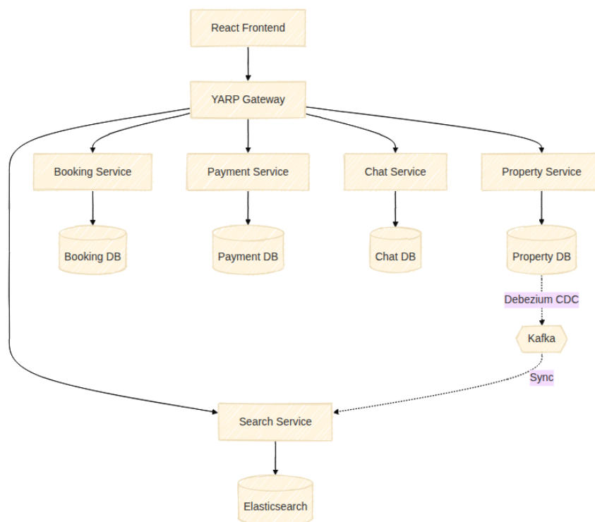
Hình 2.2. Sơ đồ Kiến trúc Tổng thể của hệ thống AirVnV
