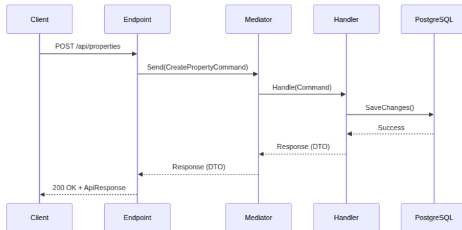
Hình 2.13. Sơ đồ Tuần tự (Sequence Diagram) minh họa luồng xử lý CQRS
