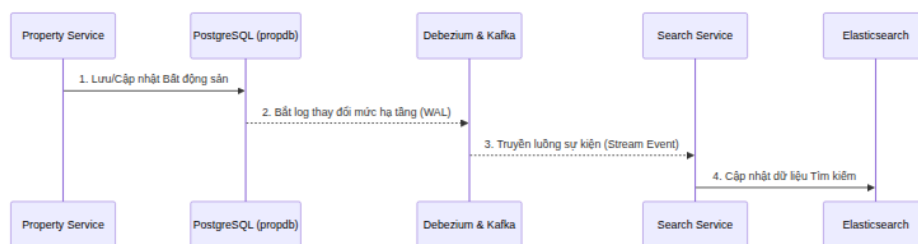
Hình 2.9. Sơ đồ Tuần tự minh họa giao tiếp Đồng bộ dữ liệu qua Kafka
