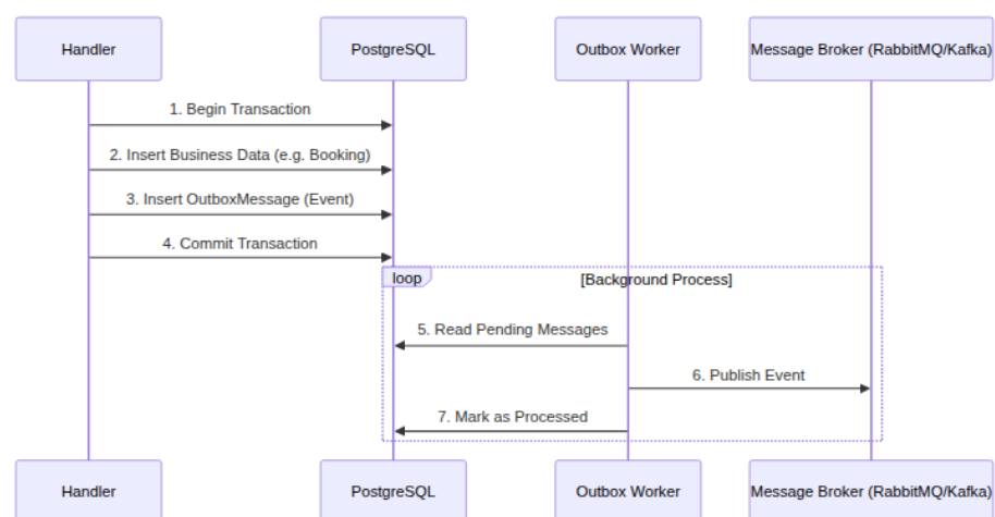
Hình 2.14. Sơ đồ Tuần tự (Sequence Diagram) cơ chế Transactional Outbox
