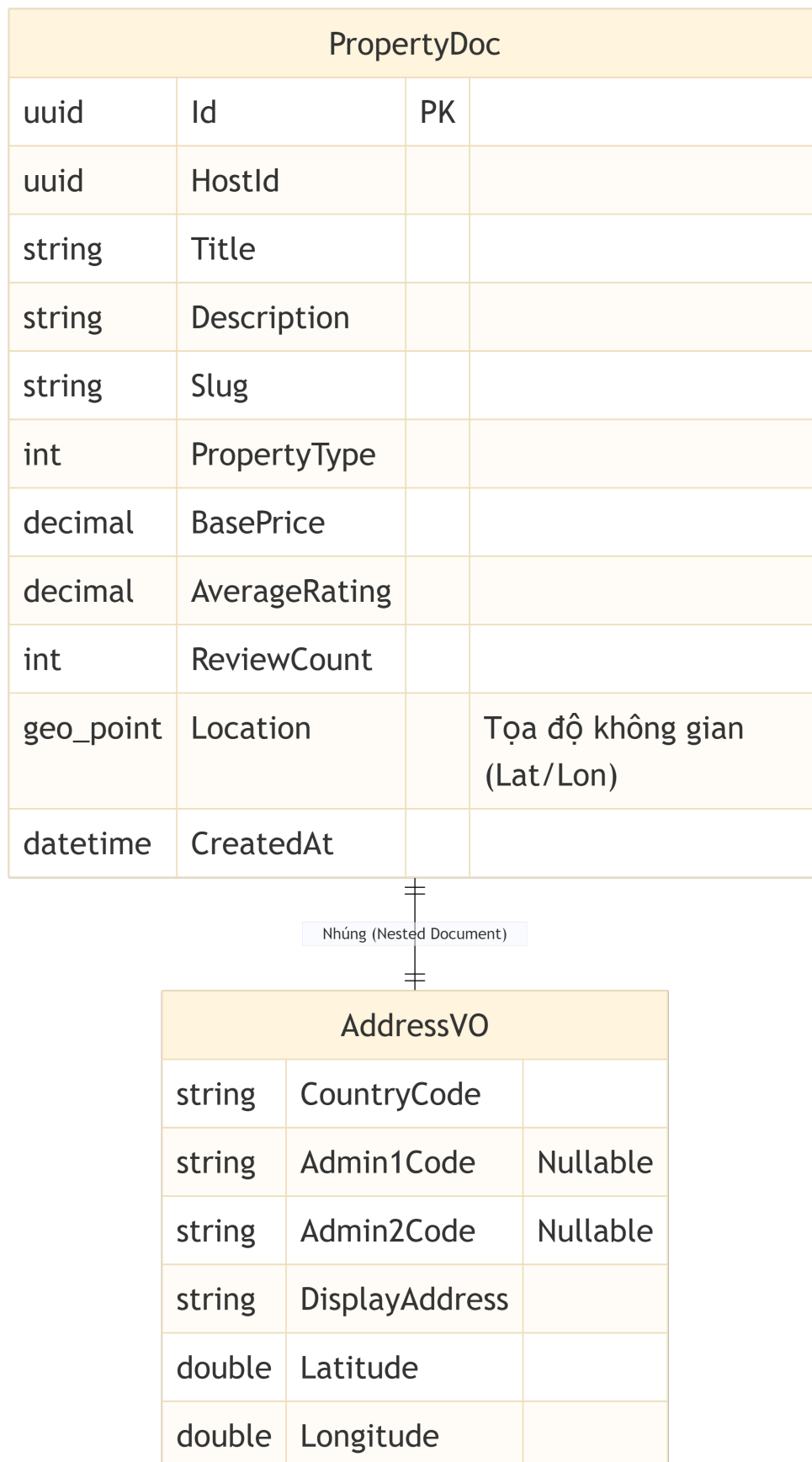
Hình 2.6. Sơ đồ Lược đồ Tài liệu (Document Schema) của Search Service
