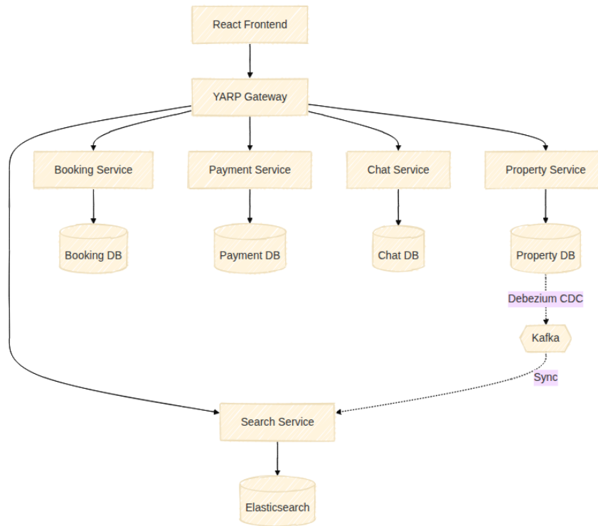
Hình 2.8. Sơ đồ Kiến trúc Tổng thể của hệ thống AirVnV
