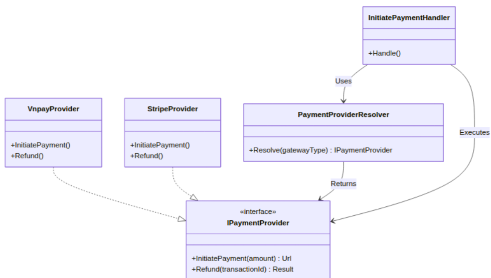
Hình 2.16. Sơ đồ Lớp (Class Diagram) mô hình Strategy Pattern tại PaymentService
