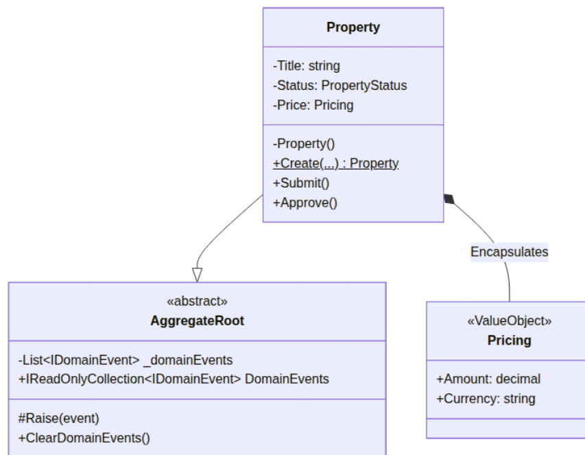
Hình 2.17. Sơ đồ Lớp (Class Diagram) mô tả Aggregate Root trong DDD
