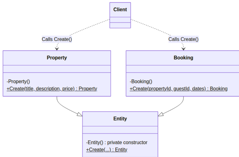
Hình 2.18. Sơ đồ Lớp (Class Diagram) của Factory Method Pattern
