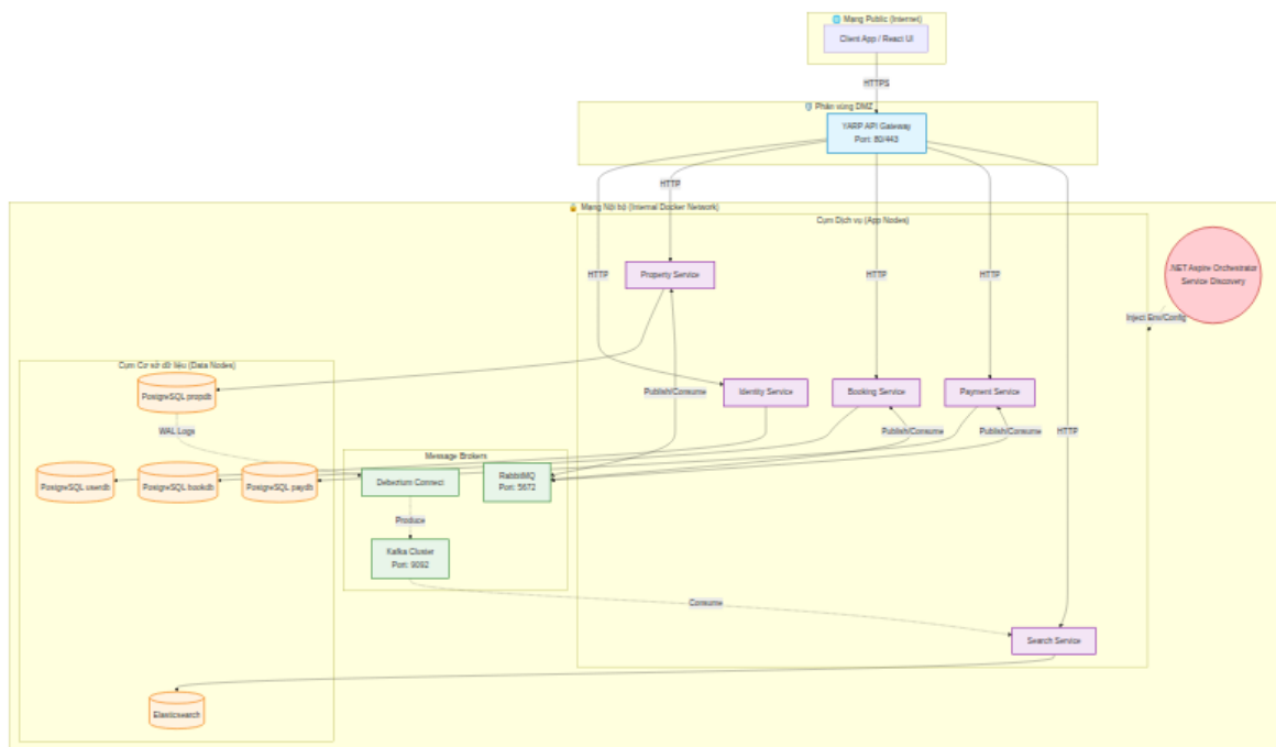
Hình 2.19. Sơ đồ Triển khai (Deployment Diagram) các Node và Phân vùng mạng
