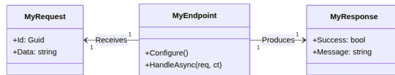
Hình 2.11. Sơ đồ Lớp (Class Diagram) cấu trúc REPR Pattern
