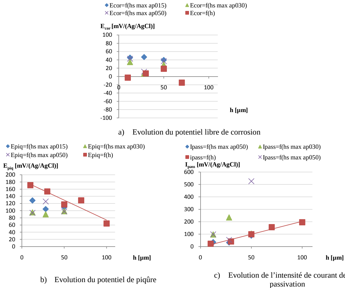
Figure 36. Evolution des paramètres électrochimiques des surfaces obtenues par tournage en superfinition : Comparaison de l'effet de h à l'effet de h_{s \max}
