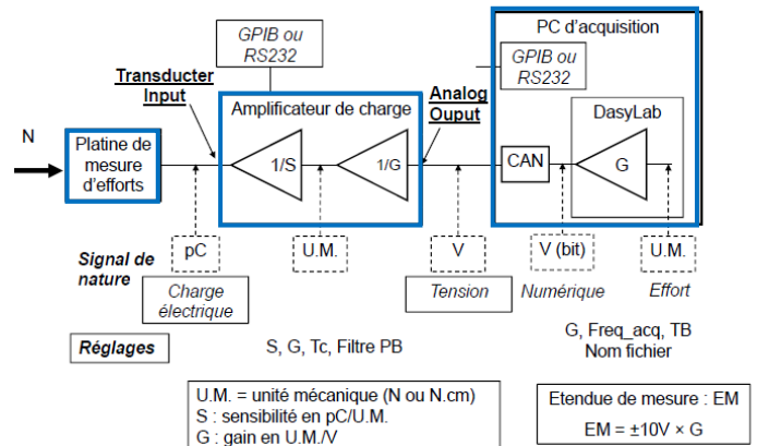
Figure 14. Synoptique du processus de mesure des efforts
