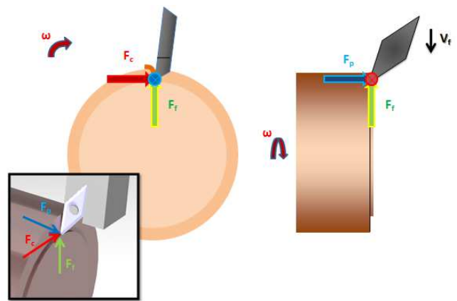
Figure 21. Efforts appliqués à l'outil
