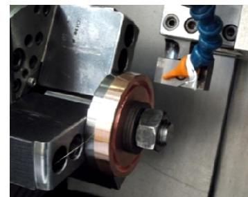
Figure 9. Montage d'essai en coupe 2D
