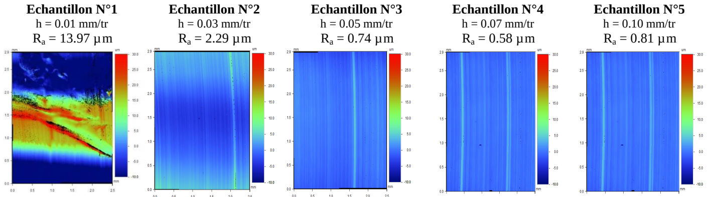
Figure 28. Impact de la coupe orthogonale sur la rugosité R_a
