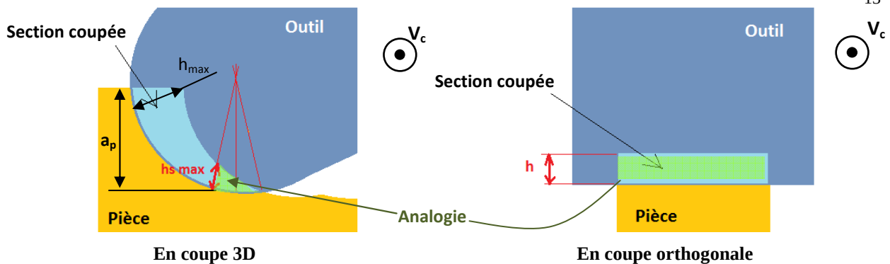
Figure 10. Comparaison entre la géométrie de coupe entre 3D et orthogonale
