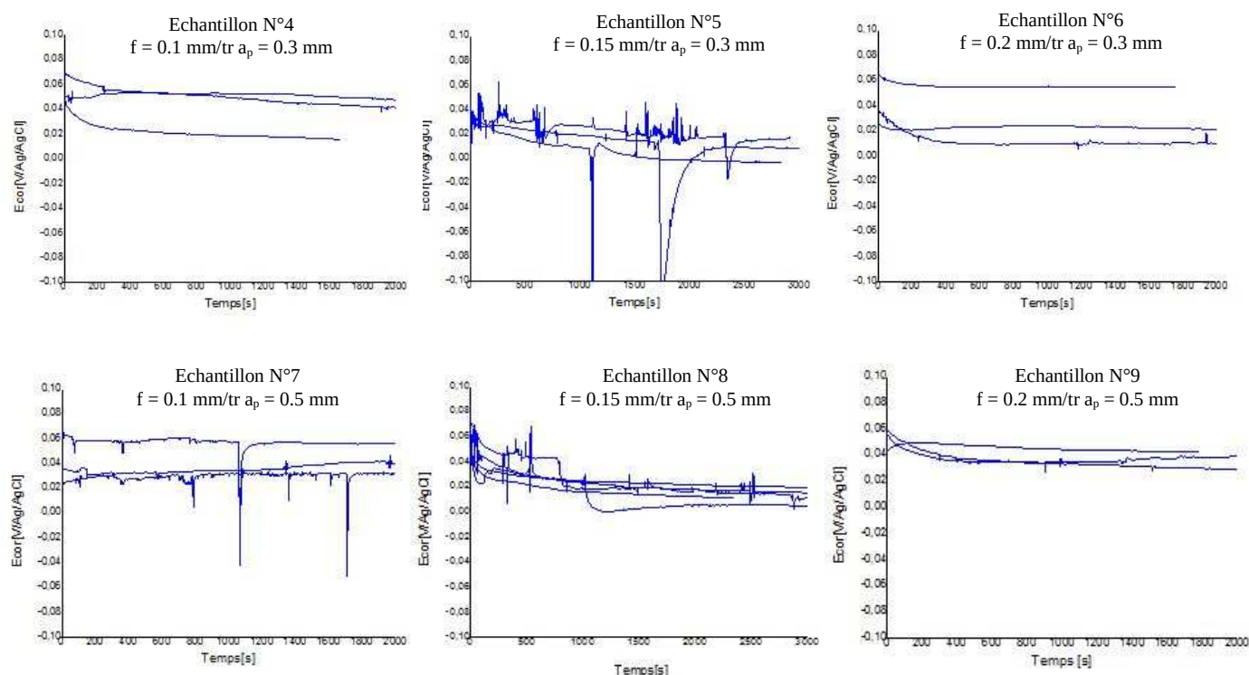
Figure 29. Evolution du potentiel libre de corrosion E_{cor} en fonction du temps sur les neuf surfaces dressées dans 1M NaClO 4 avec capillaire de Ø300 µm
