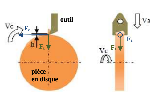
Figure 1.b. Déroulage de disque
