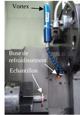
Figure 5. Montage de l'essai en coupe 3D
