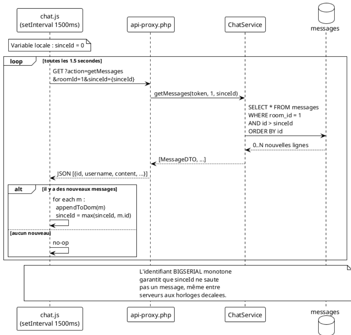
FIGURE 8 – Séquence du polling de messages côté navigateur (1,5 s).
