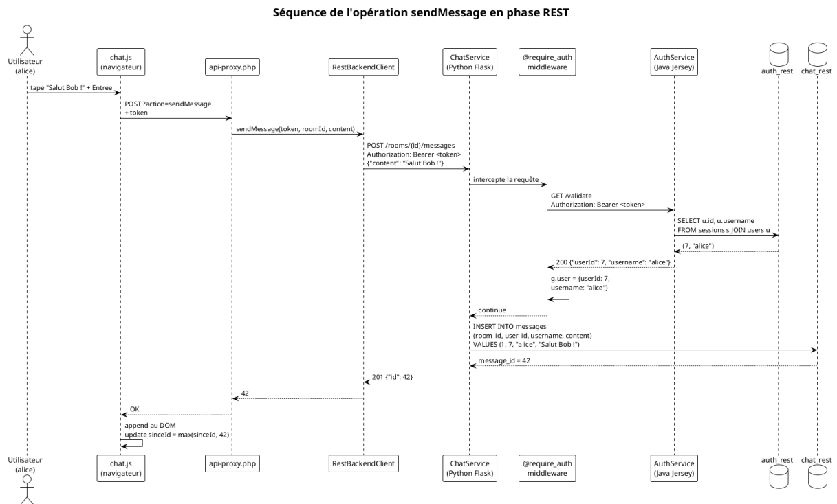
FIGURE 7 – Séquence d'un envoi de message en phase REST.
