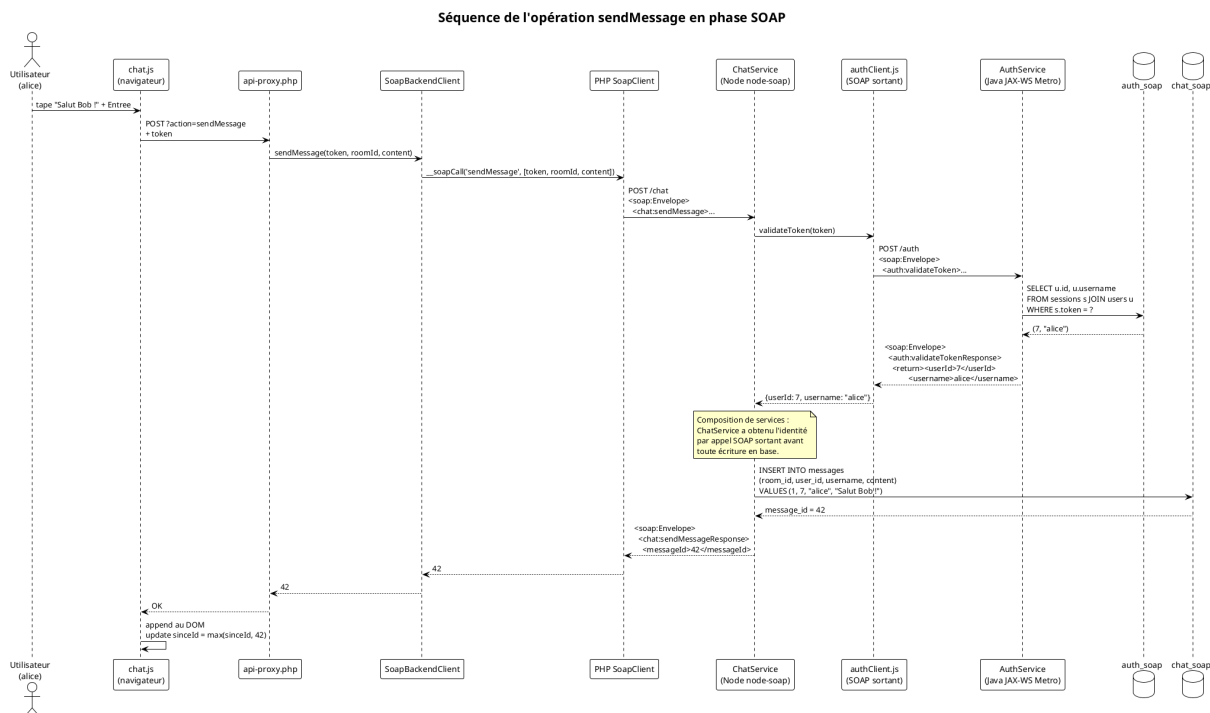
FIGURE 6 – Séquence d'un envoi de message en phase SOAP.
