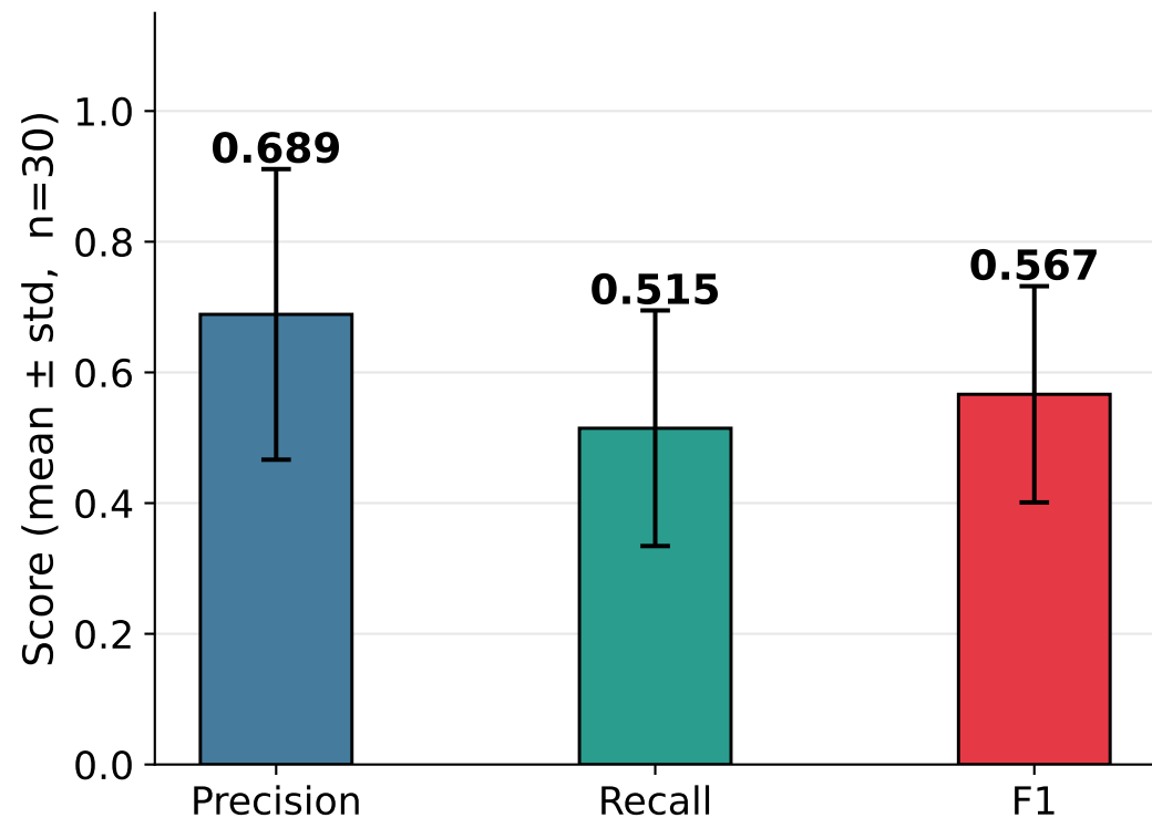
Mechanism-F1 Extractor Precision / Recall / F1
