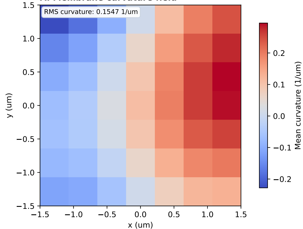
A. Membrane curvature field
