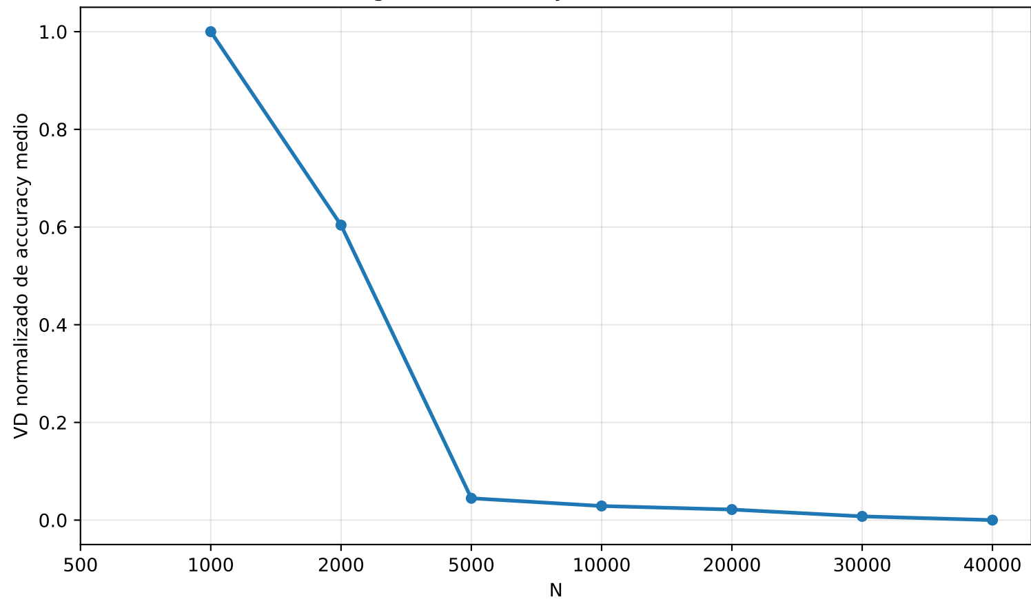
Beneficio marginal de accuracy medio medio usando fit time
