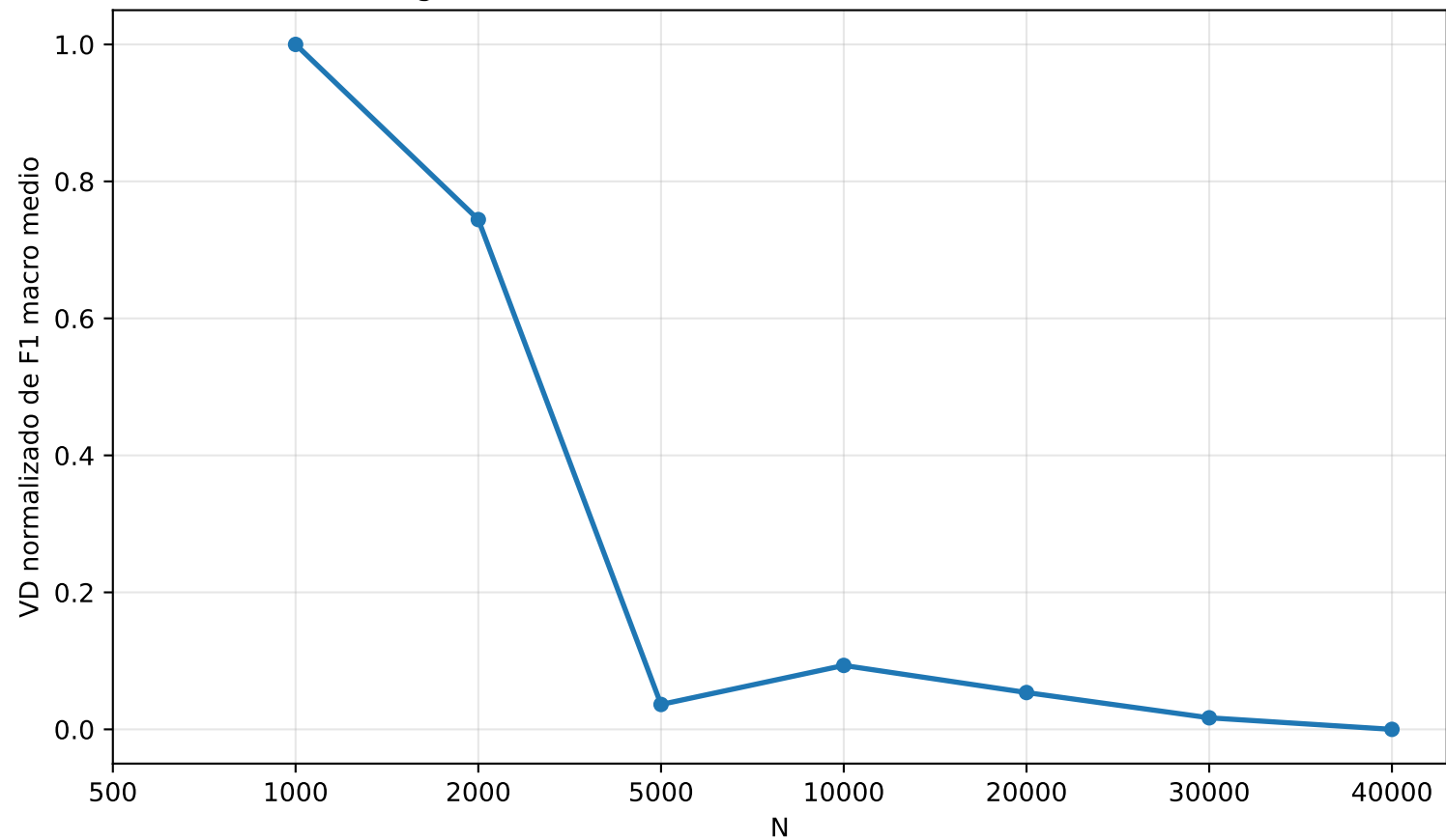
Beneficio marginal de F1 macro medio usando fit time + score time
