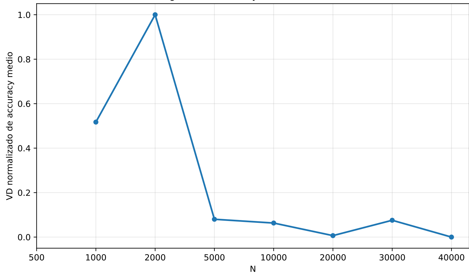
Beneficio marginal de accuracy medio usando fit time
