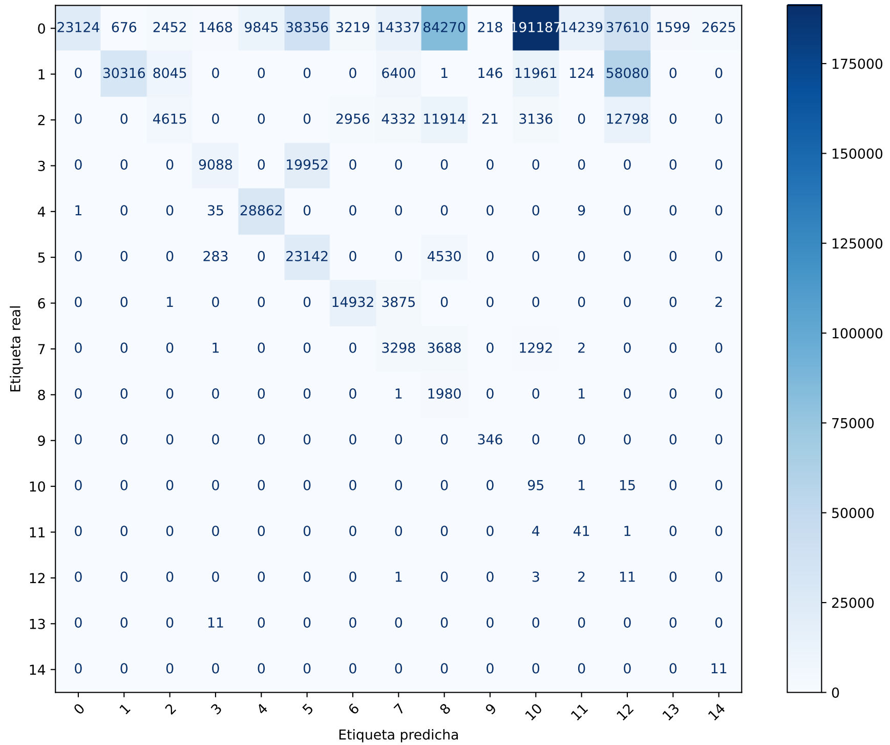
Matriz de confusion - hold-out
