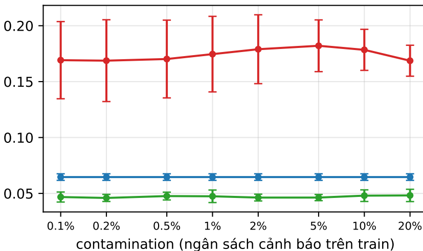
PR-AUC
