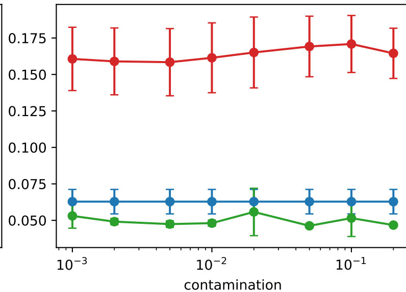
PR-AUC
