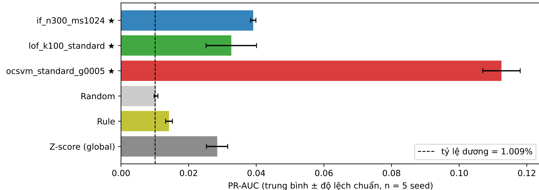
PR-AUC theo cấu hình — ★ = cấu hình tốt nhất của mô hình
