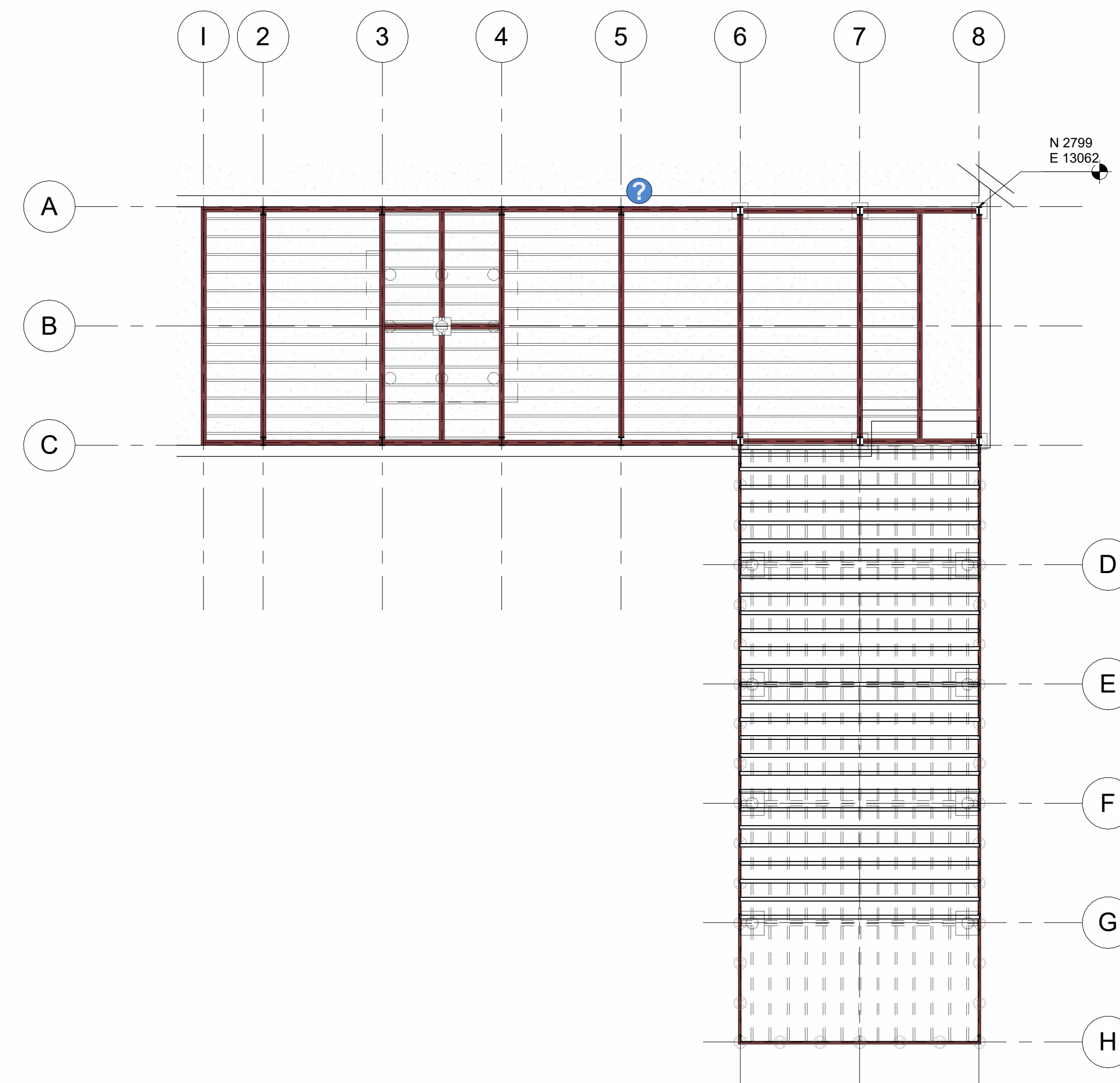
2 Level 2 1 : 100
