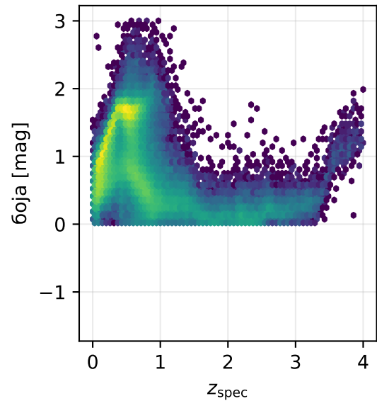
g - r
