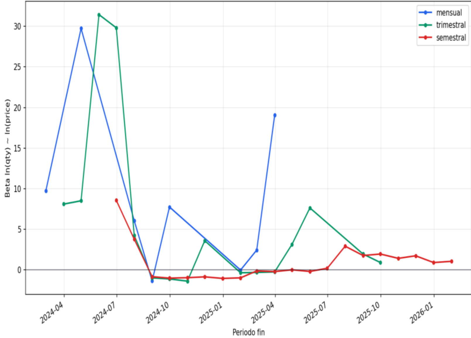
Elasticidad dinamica beta - SKU 50062267
