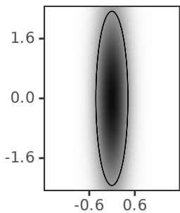
Phase-Space
