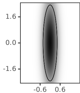
Wigner Phase-Space
