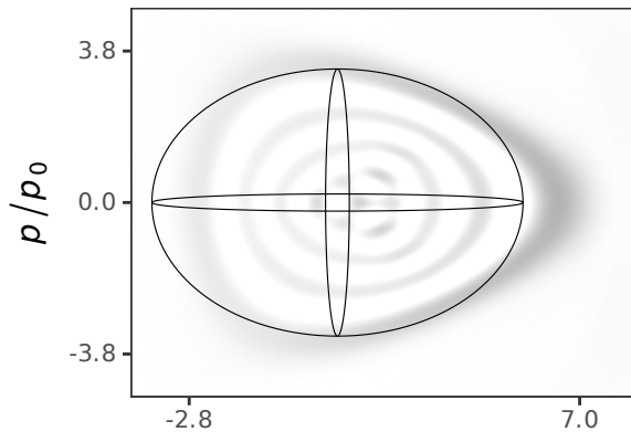
Morse n=8 (min=-0.066)
