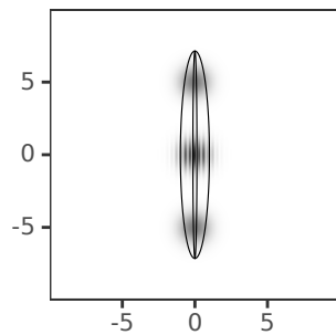
Wigner Phase-Space
